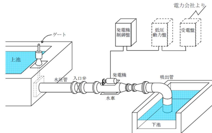
小水力発電の導入イメージ [2]
