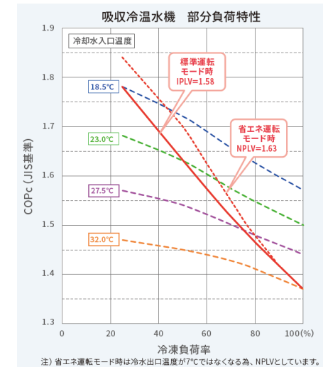
冷温水発生器 [3]
