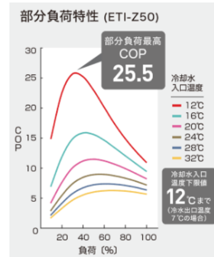
ターボ冷凍機 [2]
