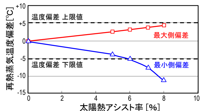
太陽熱アシスト率上限値の評価
