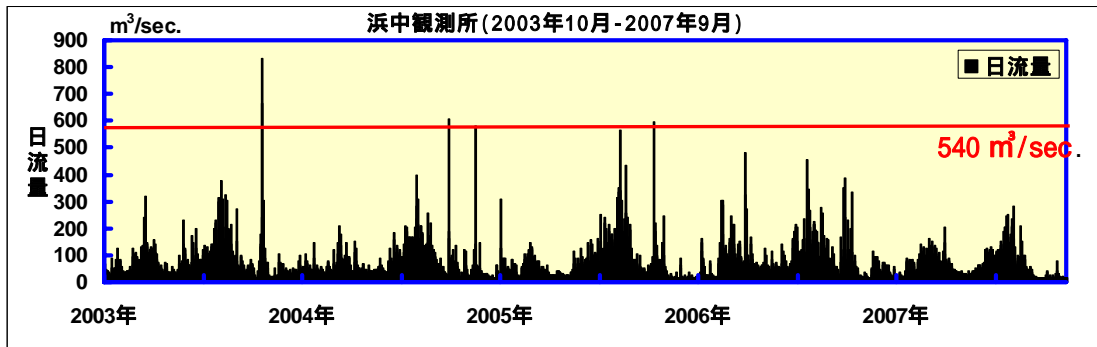
図 3.6-1 5 年間の日流量の時間変動
