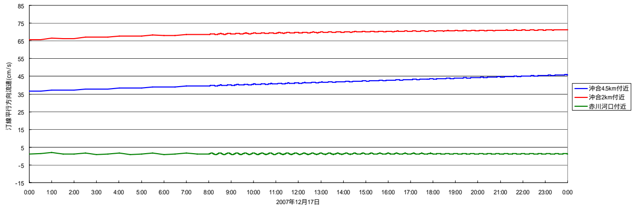
图 5.2-7 汀線平行方向(NNE)流速時系列
