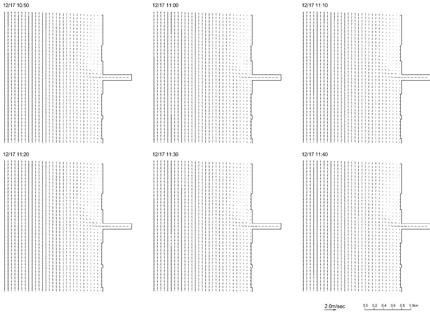
図 5.2-8(3) 赤川河口付近の流速ベクトル分布
