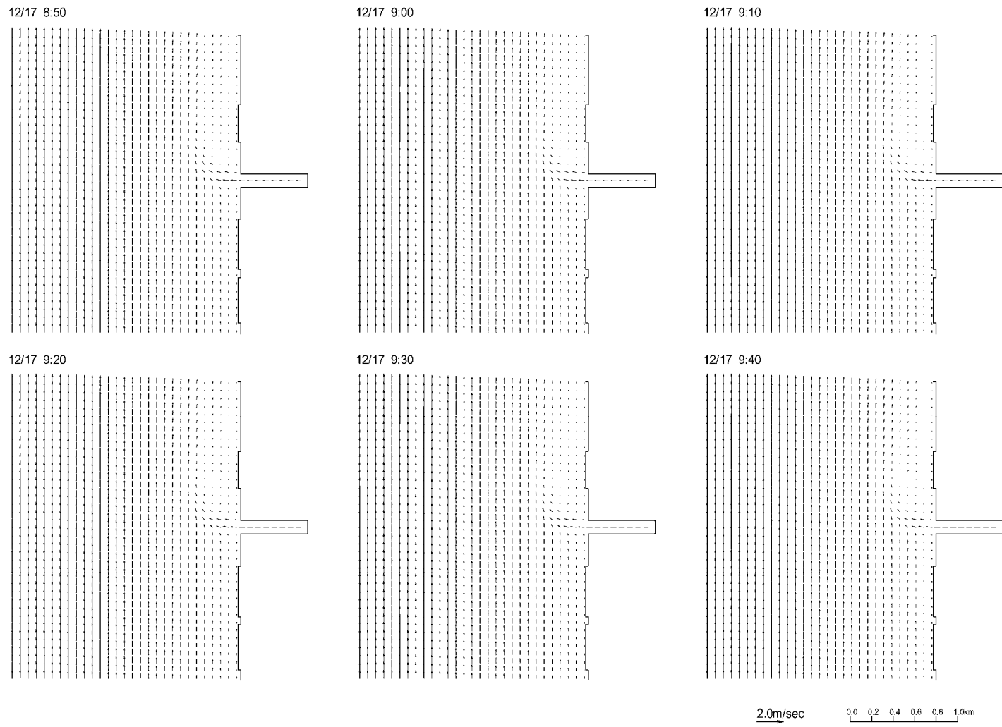
図 5.2-8(1) 赤川河口付近の流速ベクトル分布
