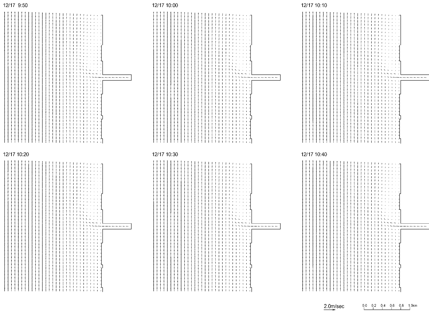
図 5.2-8(2) 赤川河口付近の流速ベクトル分布
