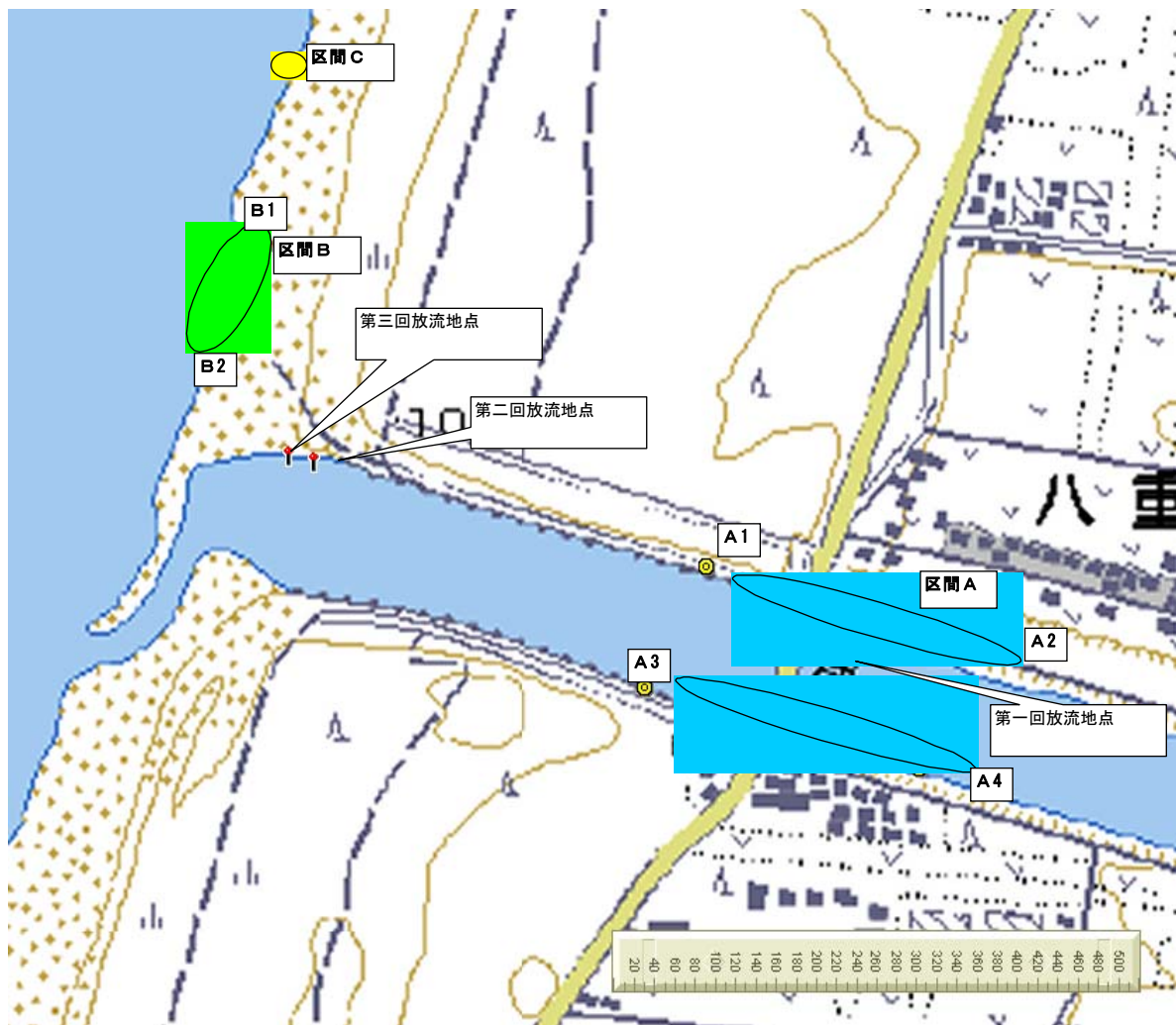
図 5.2-10 放流試験の実施位置
