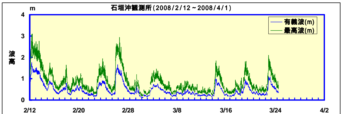
図 4.3-10(3) 風速（北西～北東のみ）及び波高の時系列（第3回～第4回）
