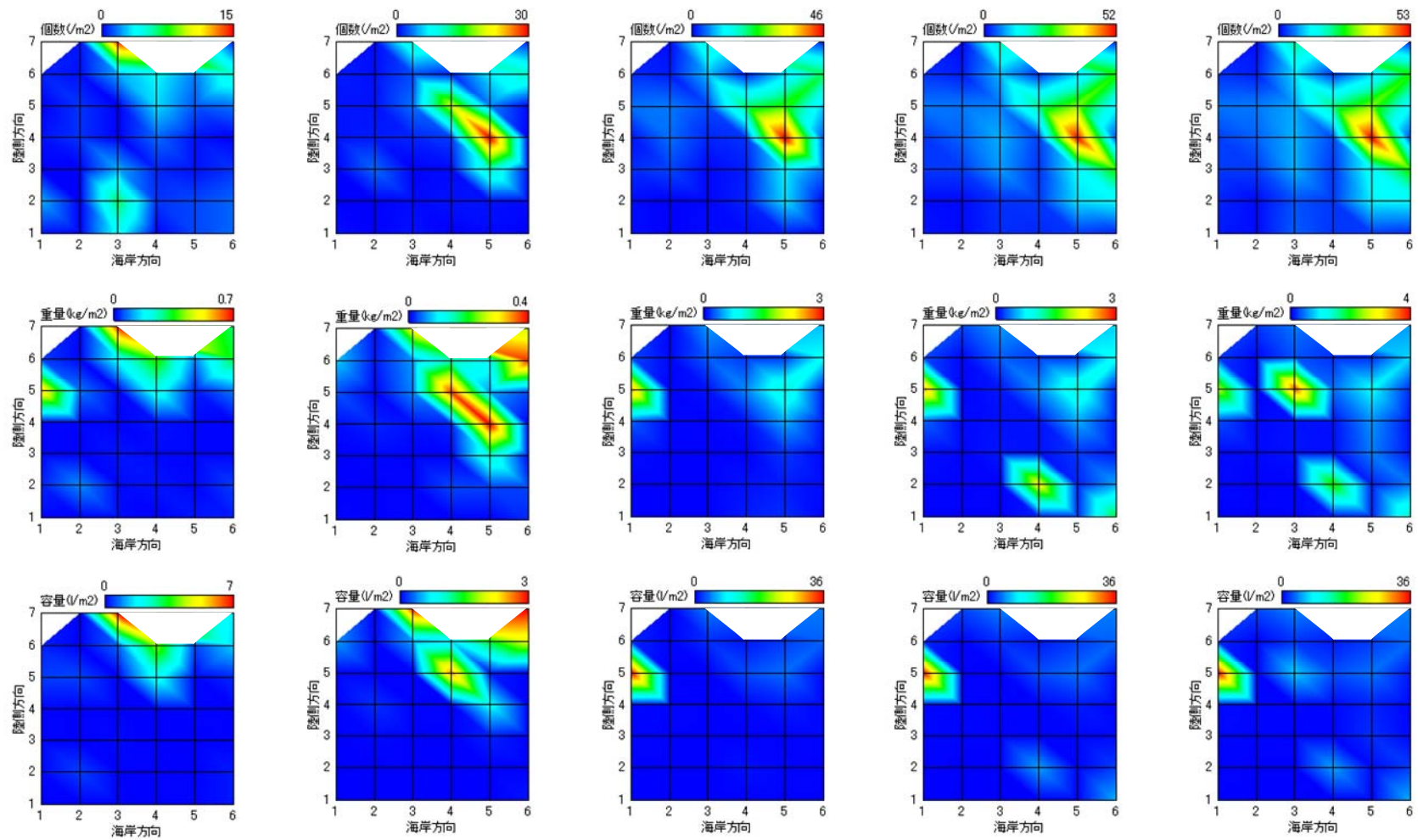
図 4.3-3 漂着ゴミの水平分布図 (各回の積算、人工物+流木・灌木)
