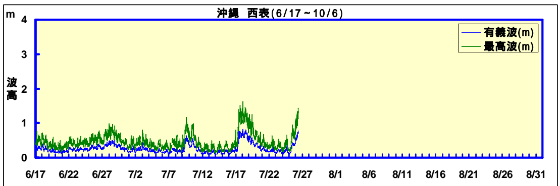
図 4.3-9(5) 風速（北西～北東のみ）及び波高の時系列（第5回～第6回）
