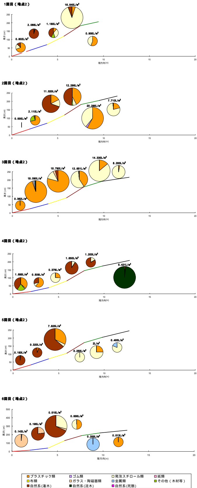
図 4.3-14(2) 地点 2 における海岸の断面形状とゴミの分布 (容量)
