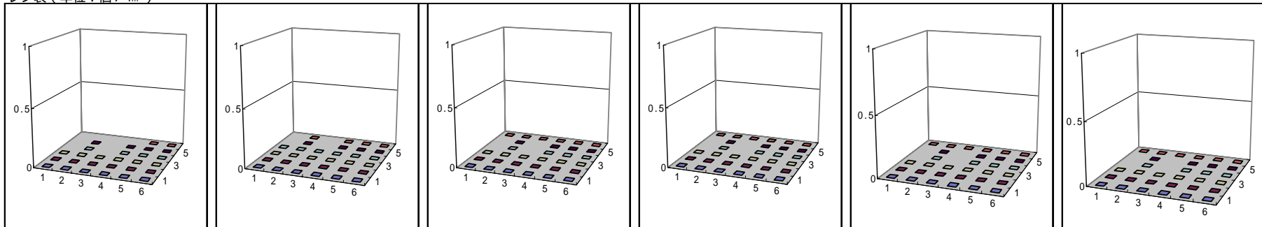
図 4.3-3(1) 漂着ゴミの種類別水平分布図 (西表島)
