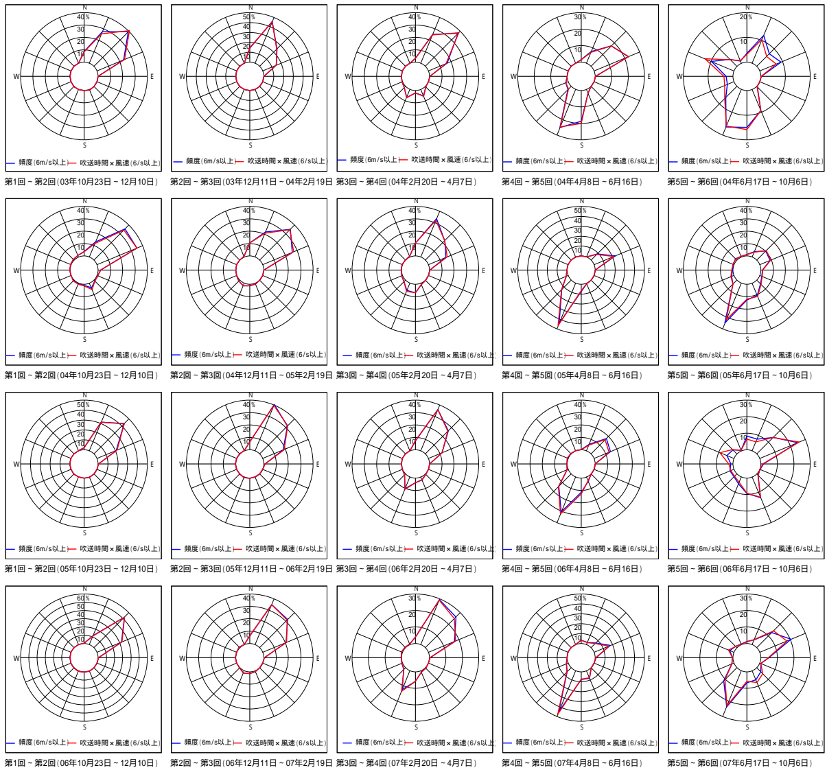
図 4.3-7 風配図及び風速 × 吹送時間 (6m/s 以上の風)
