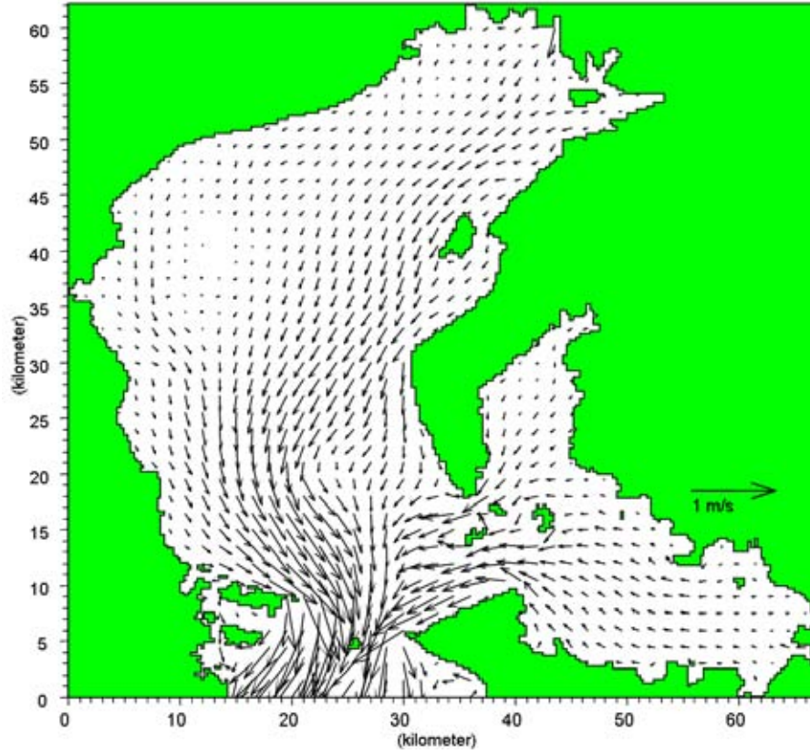
図 5.3-17 小潮期間の流出最強時の流れの水平分布図
