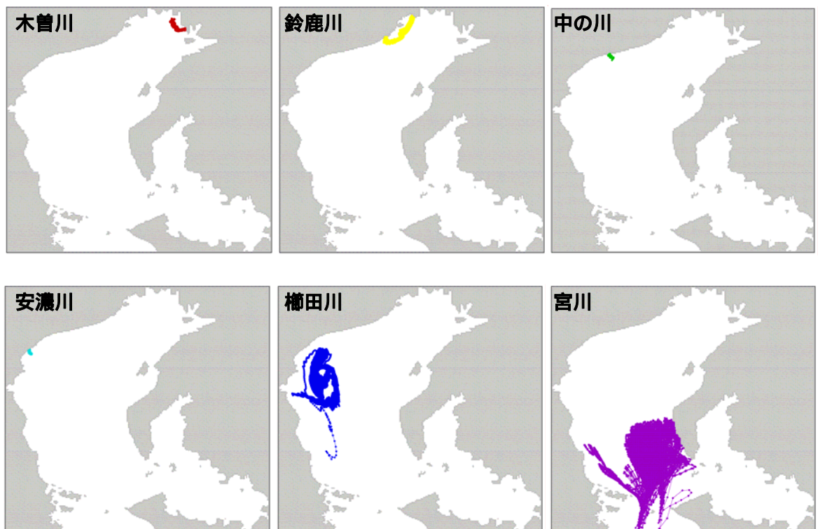
図 5.3-22 ペットボトルを対象とした漂流経路の計算結果
