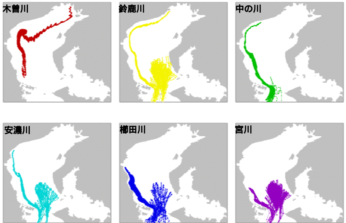
図 5.3-23 風の影響なしのケースの計算結果
