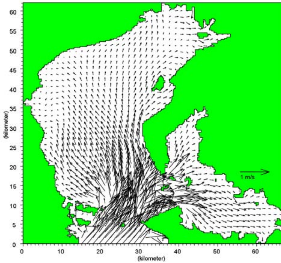
図 5.3-18 大潮期間の流入最強時の流れの水平分布図
