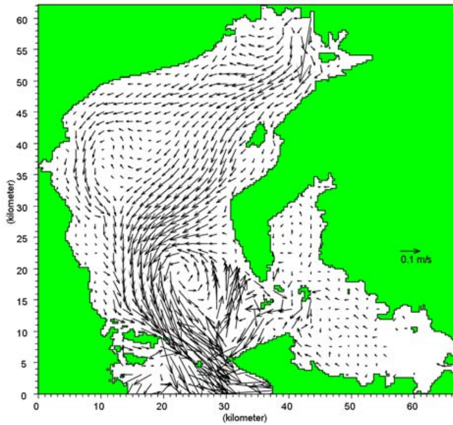
図 5.3-20 20日間平均した流速の水平分布図
