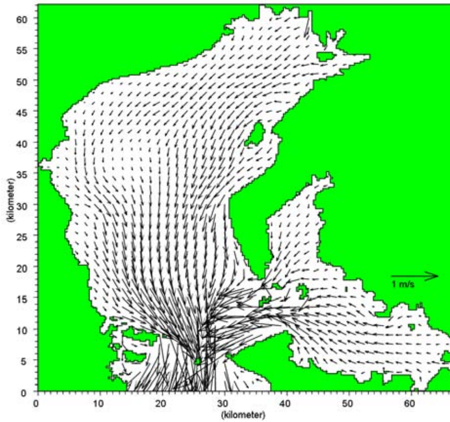
図 5.3-19 大潮期間の流出最強時の流れの水平分布図
