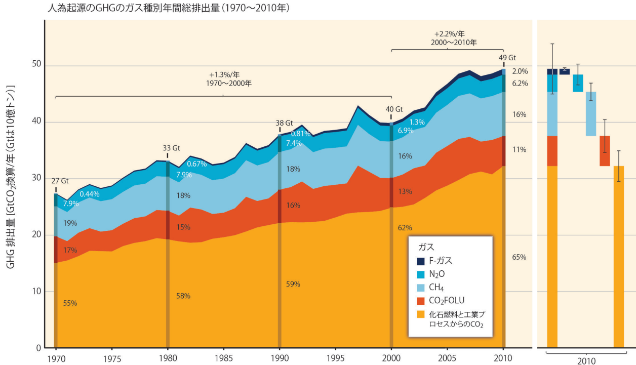
図 SPM.1 | 1970～2010 年における人為起源の GHG 排出のガス種別の年間総排出量の推移(GtCO 2 換算/年、Gt は 10 億トン)：化石燃料燃焼及び工業プロセス由来の CO 2 、林業・その他土地利用(FOLU)由来の CO 2 、メタン(CH 4 )、一酸化二窒素(N 2 O)、京都議定書の規定に含まれるフッ素化ガス(F-ガス)。2010 年の GHG 排出は、図の右側に要素ごとに分解して、エラーバーで示される不確実性(90%の信頼区間)とともに示されている。人為起源の GHG 年間総排出量の不確実性は、第 5 章(5.2.3.6)の個別のガス種ごとの推定値に基づいている。化石燃料燃焼由来の世界の CO 2 総排出量の不確実性は 8%以内である(90%の信頼区間)。FOLU 部門からの CO 2 排出には±50%程度の大きな不確実性がある。CH 4 、N 2 O、F-ガスの世界の排出量の不確実性は、それぞれ 20%、60%、20%と推定されている。2010 年は、本報告書で扱っているデータ期間における不確実性の評価が完遂され、全てのガスについて排出統計がとられている直近の年である。排出量は全て、IPCC 第 2 次評価報告書の GWP 100 128 を基に相当する CO 2 量に換算されている。FOLU 部門からの排出量データは、森林・泥炭火災と泥炭分解からの土地ベースの CO 2 排出量を表し、この報告書の第 11 章で述べられている FOLU 部門からの正味の CO 2 フラックスに近似している。期間毎の平均増加率は括弧を用いて目立つように示している。[図 1.3、図 TS.1]
