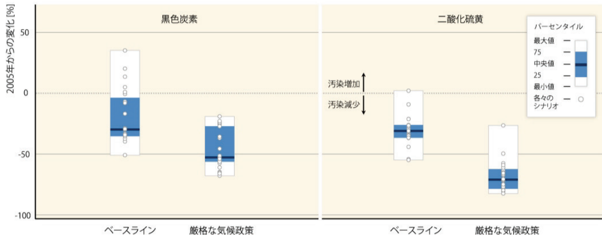
図 SPM.6 | 2005 年と比較した 2050 年の黒色炭素(BC)と二酸化硫黄(SO 2 )に対する大気汚染物質排出水準(2005 年を 0 とする)。現在、置かれている水準以上に GHG 排出を削減する努力をしないベースラインシナリオと 2100 年までに約 450 から 500(430～530)ppm CO 2 換算に達することと整合している厳格な緩和政策が比較されている。[図 6.33]
