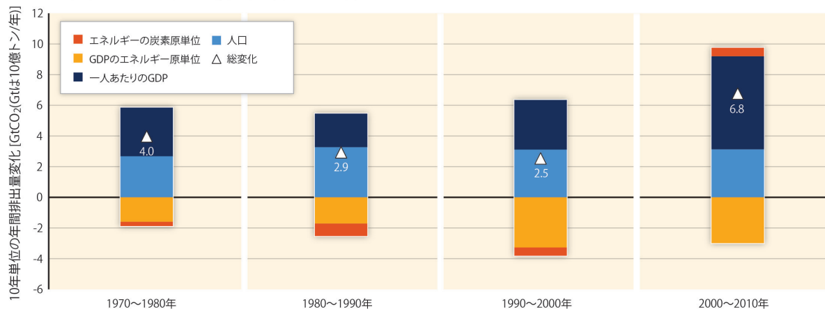
図 SPM.3 | 10 年毎の化石燃料燃焼由来の CO 2 年間総排出量変化の要因分解：人口、1 人あたりの所得(GDP)、GDP のエネルギー原単位、及びエネルギーの炭素原単位の 4 つの駆動要因に分解。棒のそれぞれの区間は、他の要因を一定に保った場合の、それぞれの要因単独での変化を表している。排出量の総変化は△で示してある。それぞれの 10 年間の排出量の変化は年当たりの Gt (10 億トン) 単位の CO 2 [GtCO 2 /年] で評価されている。所得は購買力平価を用いて、共通単位に変換した。[図 1.7]
