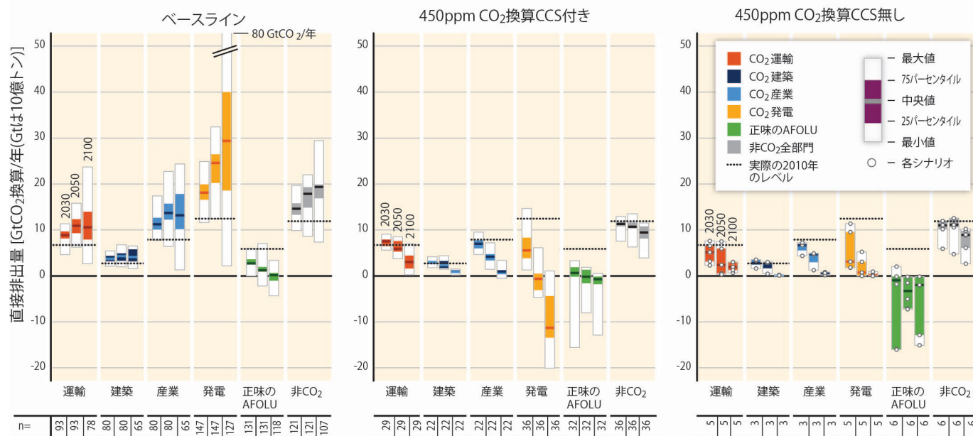
図 SPM.7 |部門別の CO 2 と全部門の CO 2 以外の GHG 類(京都議定書規定のガス)の直接排出量。ベースライン(左図)、CCS を用いて 450(430~480) ppmCO 2 換算に達する緩和シナリオ(中央の図)、同 CCS 無し(右図)。グラフの下に数字はその範囲に含まれるシナリオの数である。部門の解像度やモデルの対象期間が異なるため、範囲が部門と期間によって異なる。CCS 無しには、ほとんどのモデルにおいて 2100 年までに 450ppmCO 2 換算濃度に到達できないことに注目。この結果、右図のシナリオの数が少なくなっている。[図 6.34 及び図 6.35]
