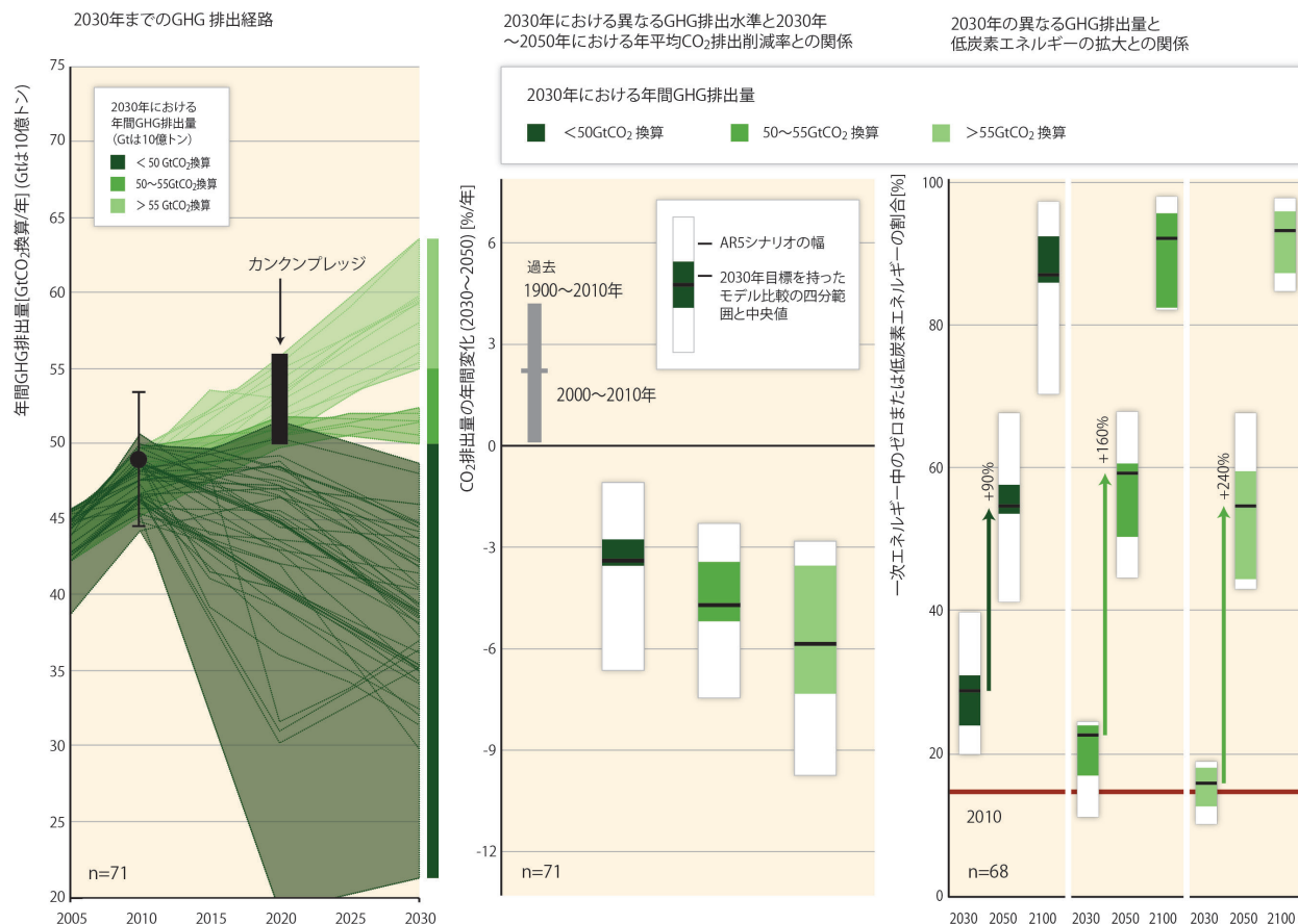
図 SPM.5 | 2100 年までに濃度が約 450 から約 500ppm(430~530ppmCO 2 換算)に達する緩和シナリオにおける、2030 年の GHG 排出水準(左図)と、2030 年から 2050 年の CO 2 排出削減率(中図)、及び 2030 年から 2050 年及び 2100 年への低炭素エネルギー拡大との関係(右図)。これらのシナリオは 2030 年までの排出水準によってグループ化されている(緑の濃さによって色分けされている)。左の図はそれぞれの 2030 年水準に達する GHG 排出量(GtCO 2 換算/年)の経路を示している。黒い棒はカンクンプレッジが意味する GHG 排出量の推定される不確実性範囲を示している。中央の図には 2030 年から 2050 年の期間の年間 CO 2 排出削減率の平均値を表示している。これは、明確な 2030 年目標を持った最近のモデル間比較におけるシナリオ間の中央値と 4 分位範囲を、WGIII AR5 のためのシナリオデータベースのシナリオ範囲と対比している。1900~2010 年の間の過去の排出量の年間変化率(20 年間変わっていない)及び 2000~2010 年の間の年間平均排出量の変化は灰色で示されている。右側の図の矢印は、2030 年のそれぞれの GHG 排出水準について、2030 年から 2050 年に向けてのゼロ及び低炭素エネルギーの供給拡大の大きさを示している。ゼロ及び低炭素エネルギー供給には、再生可能エネルギー、原子力エネルギー、二酸化炭素回収・貯留(CCS)付きの化石燃料、及び CCS 付きのバイオエネルギー(BECCS)などがある。注:シナリオのうち、使用モデルにおいて完全に制限のない緩和技術ポートフォリオが使われた場合(初期設定技術の仮定)のものだけを示している。シナリオのうち、正味の負の排出が大きい(>20GtCO 2 /年)もの、外部起因の炭素価格仮定を用いているもの、及び 2010 年の排出が明らかに過去の幅からはみ出るものは除いてある。右側の図では 68 のシナリオのみが用いられている。図に示した 71 シナリオのうち 3 つにゼロ-及び低炭素-エネルギーの割合の計算に必要な一次エネルギーのいくつかの細区分の報告がないためである。[図 6.32, 図 7.16, 13.13.1.3]
