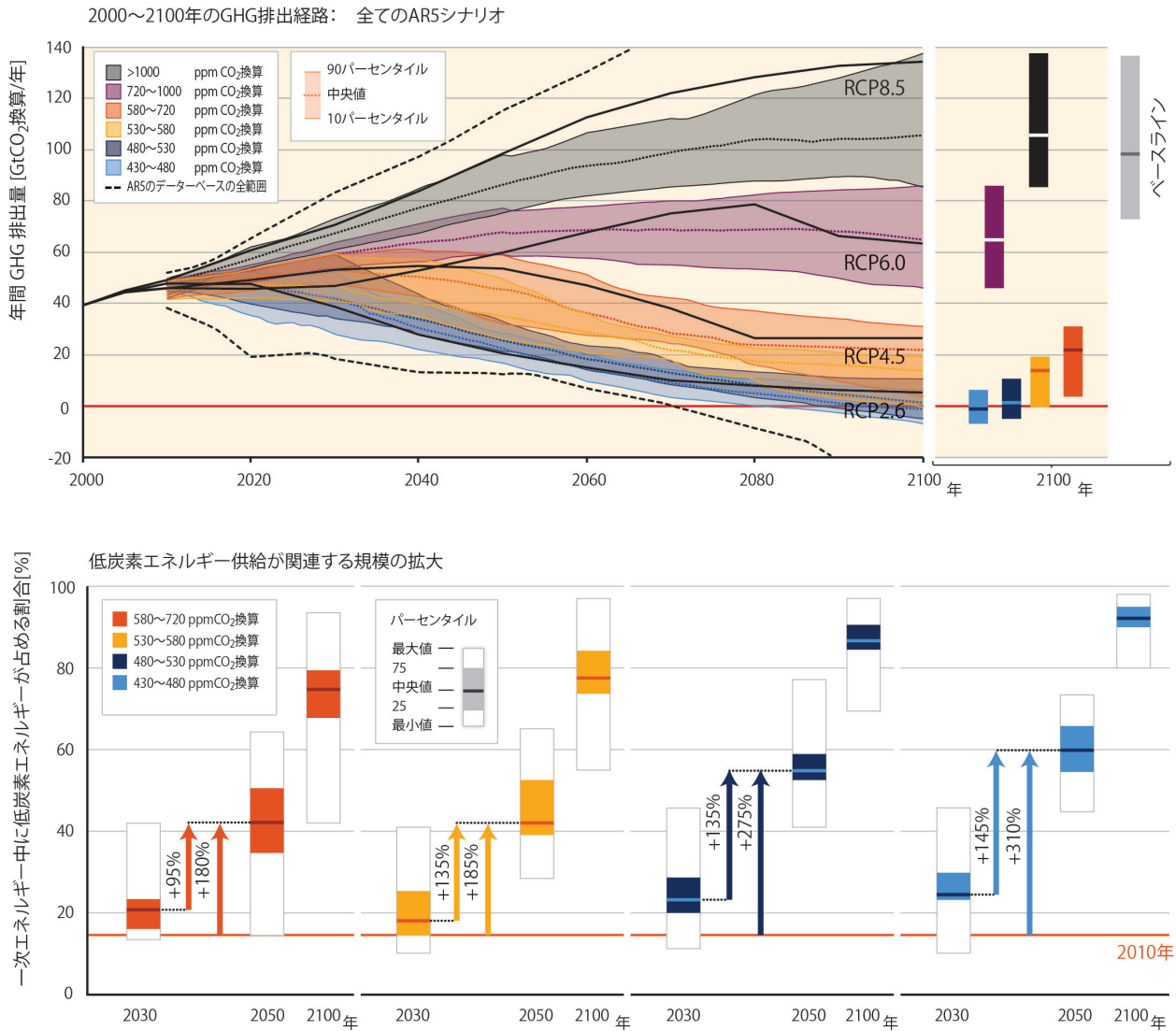
図 SPM.4 | ベースライン及び異なる長期の濃度水準に対する緩和シナリオにおける、世界の GHG 排出量(GtCO 2 換算/年、Gt は 10 億トン)の経路(上図)[図 6.7]、及び 2030 年、2050 年、2100 年での関連する低炭素エネルギーの 2010 年水準からの必要な拡大量(一次エネルギーに占める%で表す) (下図)。[図 7.16] 下の図は、技術の利用に制限があるシナリオと炭素価格の経路を外生的に与えるシナリオを除外している。CO 2 換算排出量と CO 2 換算濃度の定義に関しては WGIIIAR5 の用語集を参照のこと。
