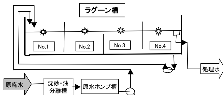
図3-2-2 炭酸飲料廃水処理装置概念図
