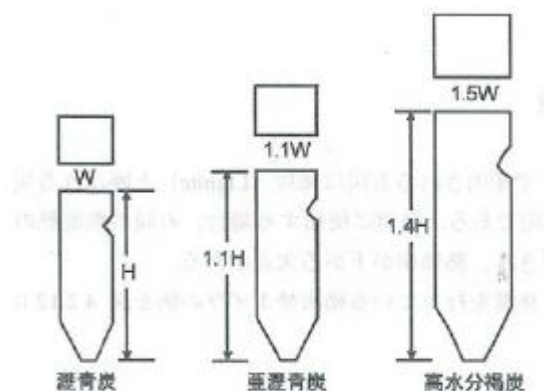
図 6.7-1 ボイラ火炉高さの比較（高水分）
