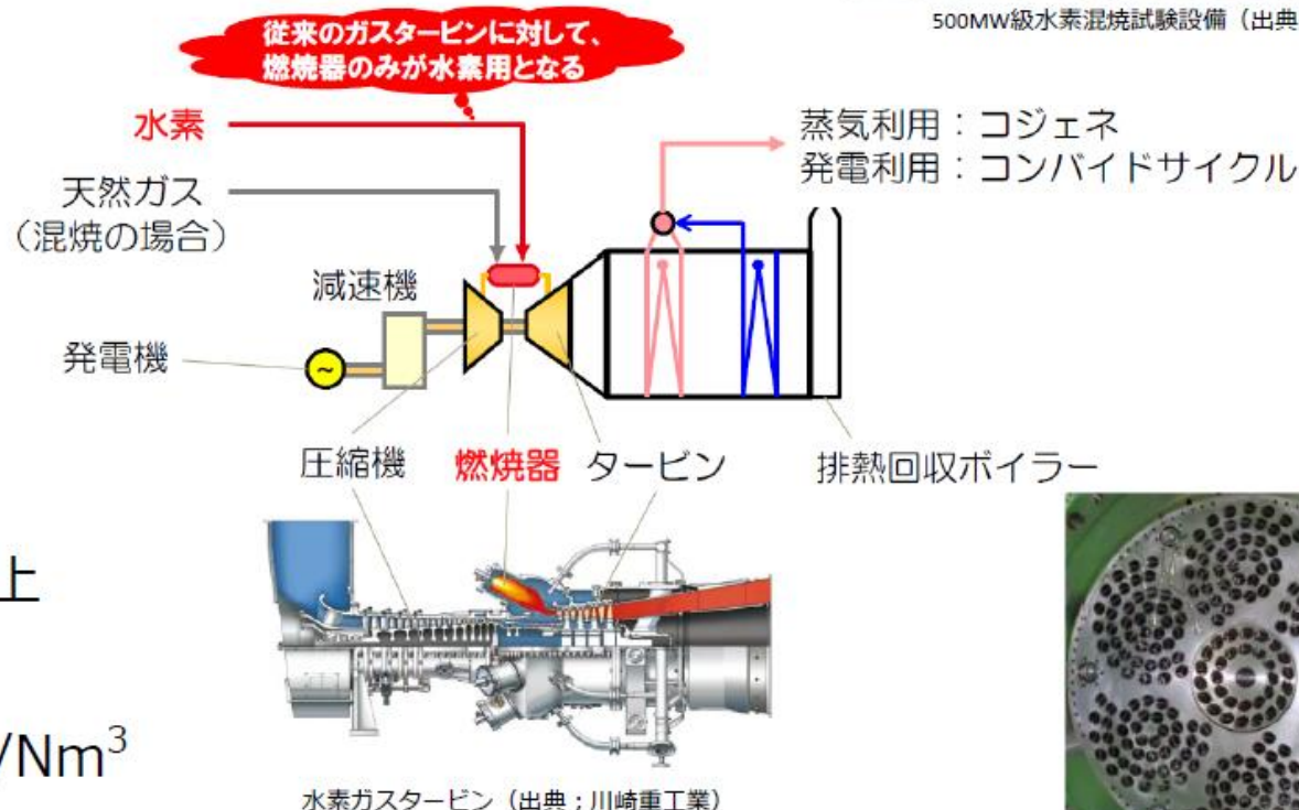
水素ガスタービン（出典；川崎重工業）
