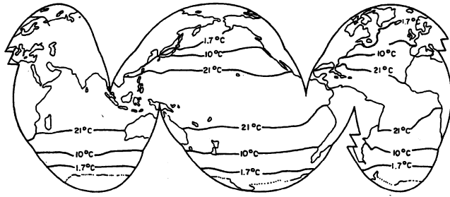
Isotheres
