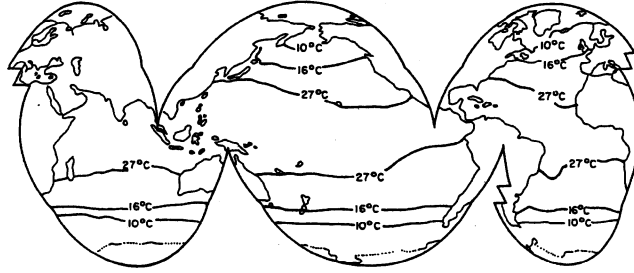
Isotheres
