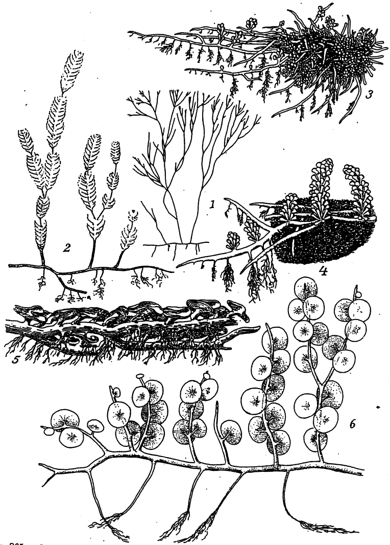
Fig. 265. Caulerpa n. REINKE, BÖRGESEN u. SVEDLIUS. 1 C. fastigiata . 2 C. crassifolia . 3. u. 4 C. racemosa . 5 C. nummularia . 6 C. macrodisca .
