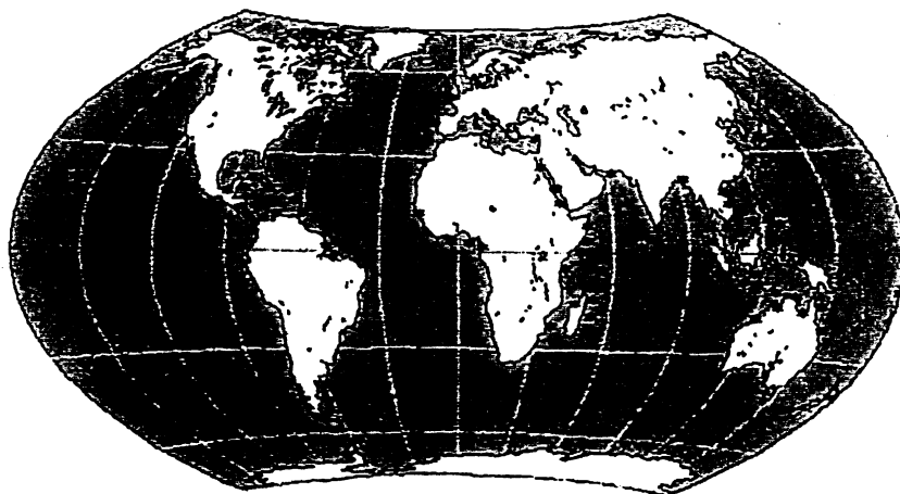
Caulerpa taxifolia イチイツタの分布
