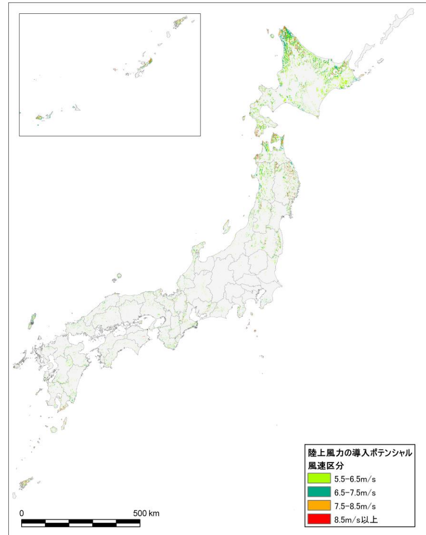
陸上風力の導入ポテンシャル分布図
