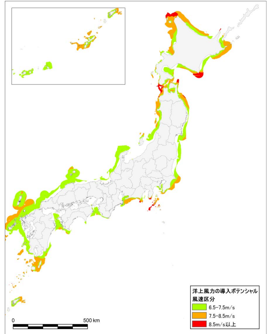
洋上風力の導入ポテンシャル分布図
