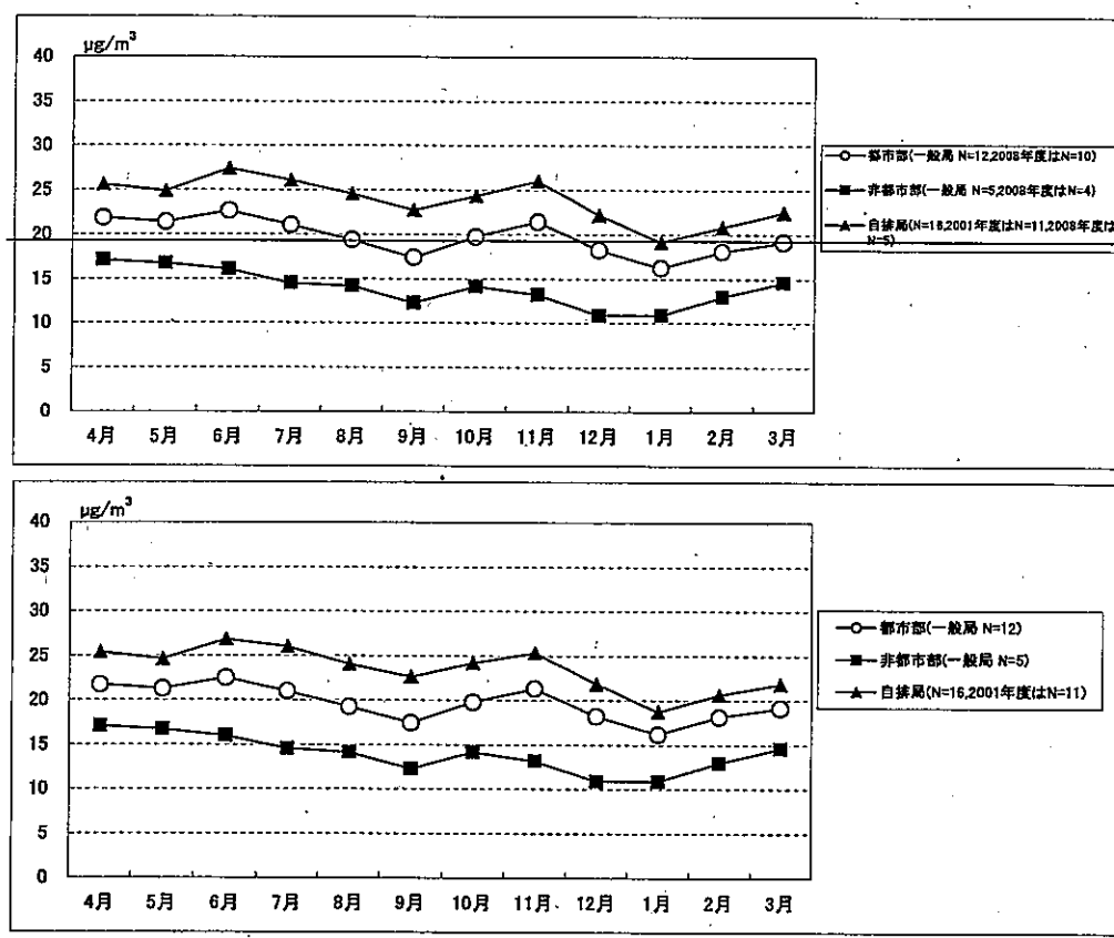
図2.1.1.2 PM 2.5 (50℃加熱方式TEOM)質量濃度の月平均値の変化 (2001～2008年度の月平均値の平均)
