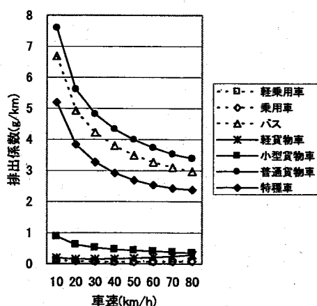
図=.4 NOx排出係数 (平成19年度、一例)
