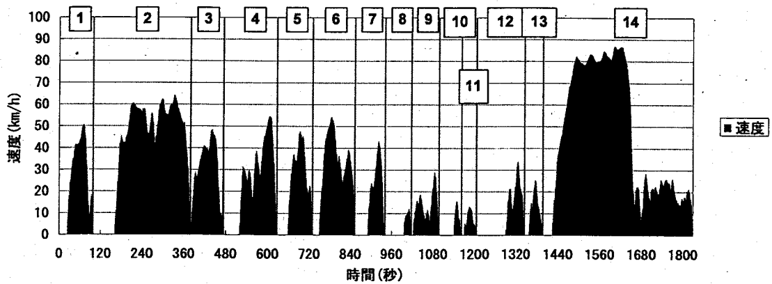
図=.3 JE05モード * の速度変化 (四角内番号が分割・集約するトリップ単位)
