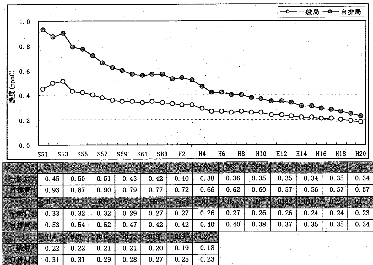
図 3-7 非メタン炭化水素濃度（午前 6 時～9 時の 3 時間平均値）の推移
