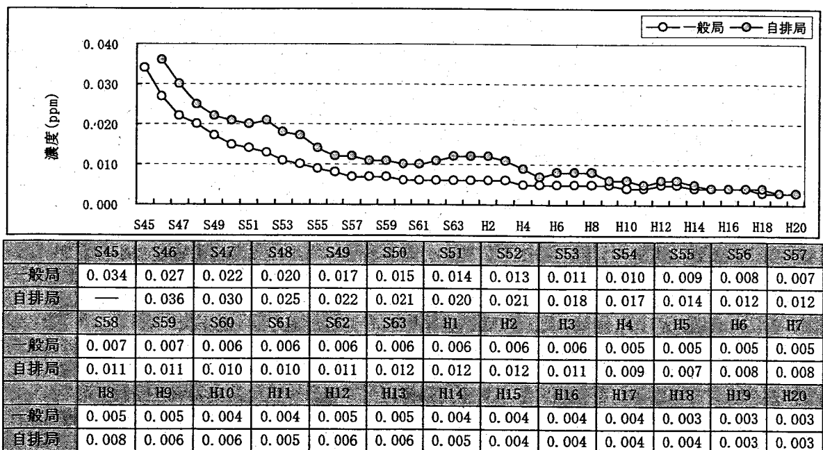
図 4-2 二酸化硫黄濃度の年平均値の推移
