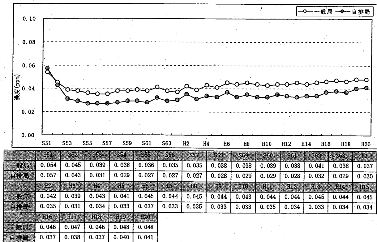
図3-2 光化学オキシダントの昼間の日最高1時間値の年平均値の推移
