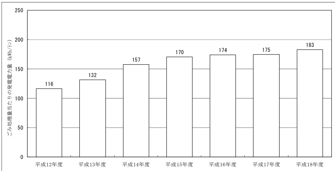
図－13 ごみ処理量当たりの発電電力量
