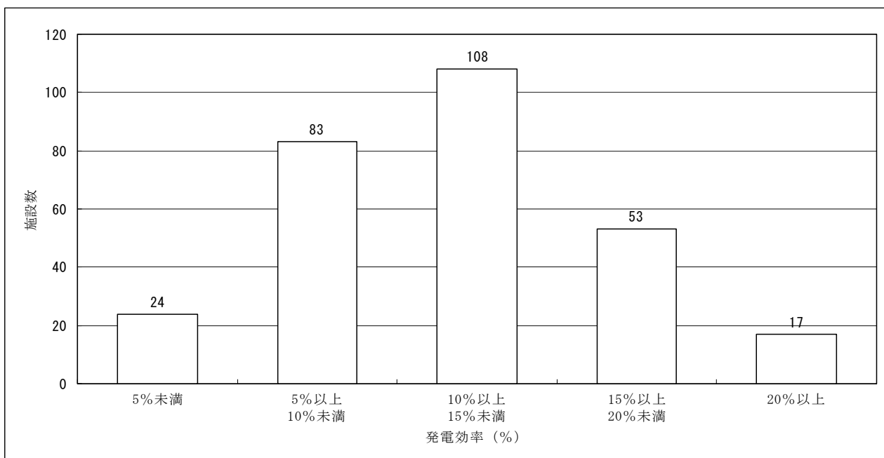
図－14 ゴミ焼却施設の発電効率別の施設数 （注12）
