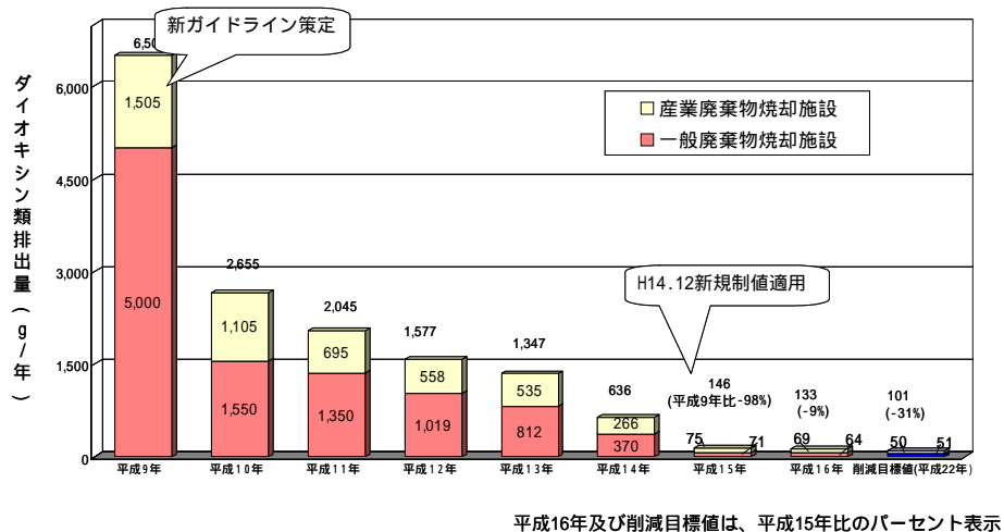
廃棄物焼却施設のダイオキシン類発生量推移
