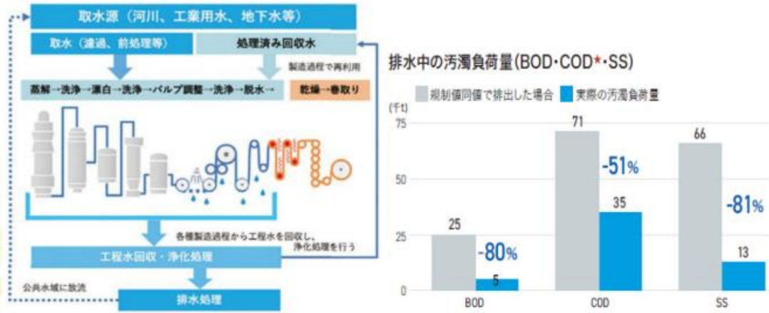
排水の循環フロー（簡易図）と排水中の汚濁負荷量
