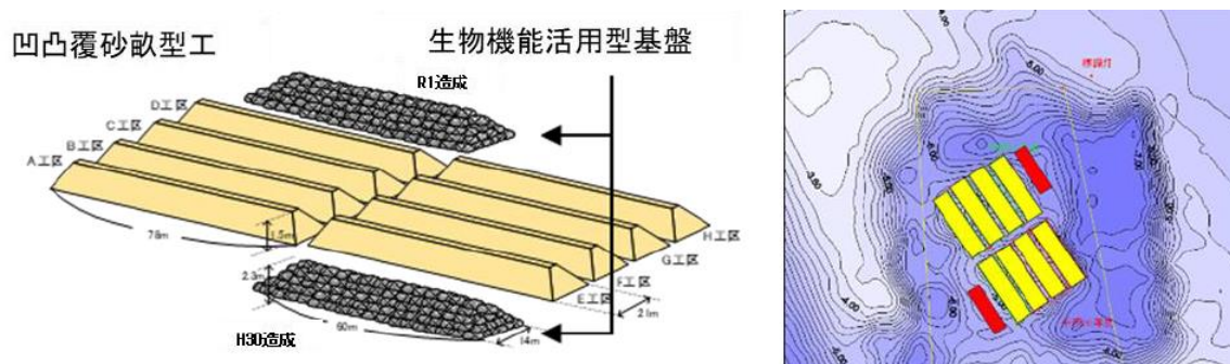
H25・H26年度凹凸覆砂畝型工+生物機能活用型基盤
