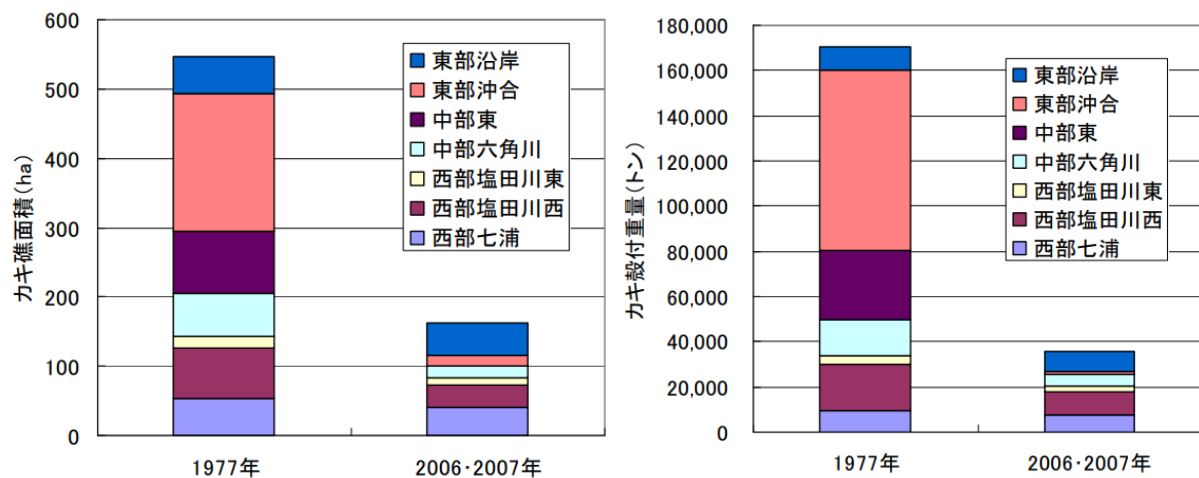
図3 カキ礁分布面積(左)とカキ生物量(右)の推計 (1977年及び2006-2007年)
