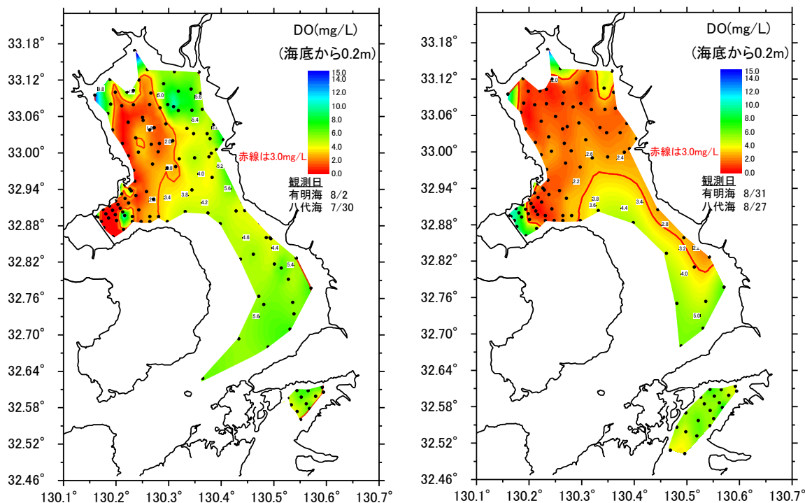
図 2 有明海及び八代海における底層溶存酸素濃度の分布 (左図:2021 年 8 月 2 日、右図:2021 年 8 月 31 日)
