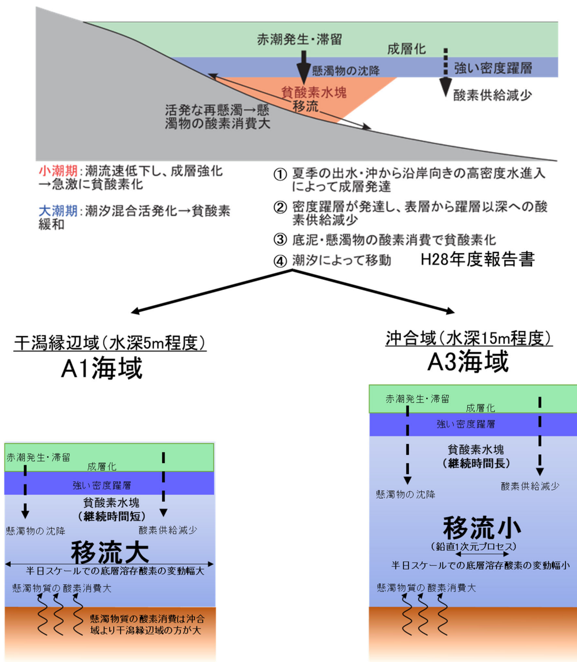
付図 3.6.2-2 有明海湾奥部における貧酸素水塊発生の模式図
