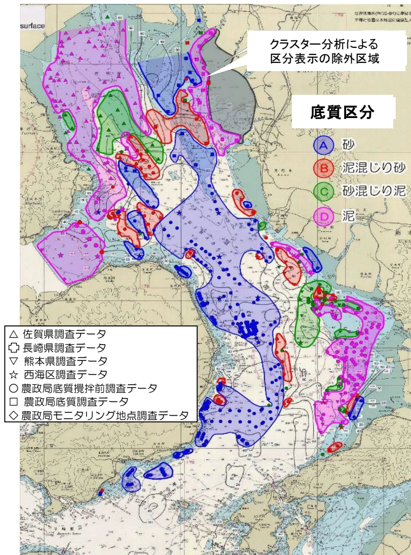
11 付図 3.5.1-3 有明海の底質特性別海底質区分図(2023 年)
