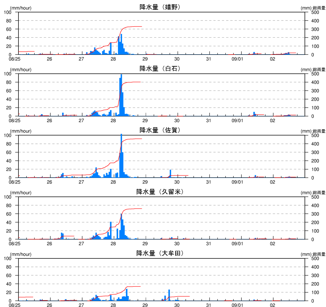
付図 3.5.1-11 降水量の経時変化
