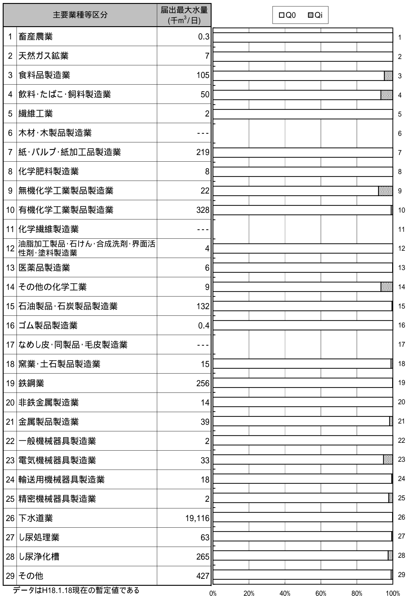
図2 3 海域計 - 窒素・りん
