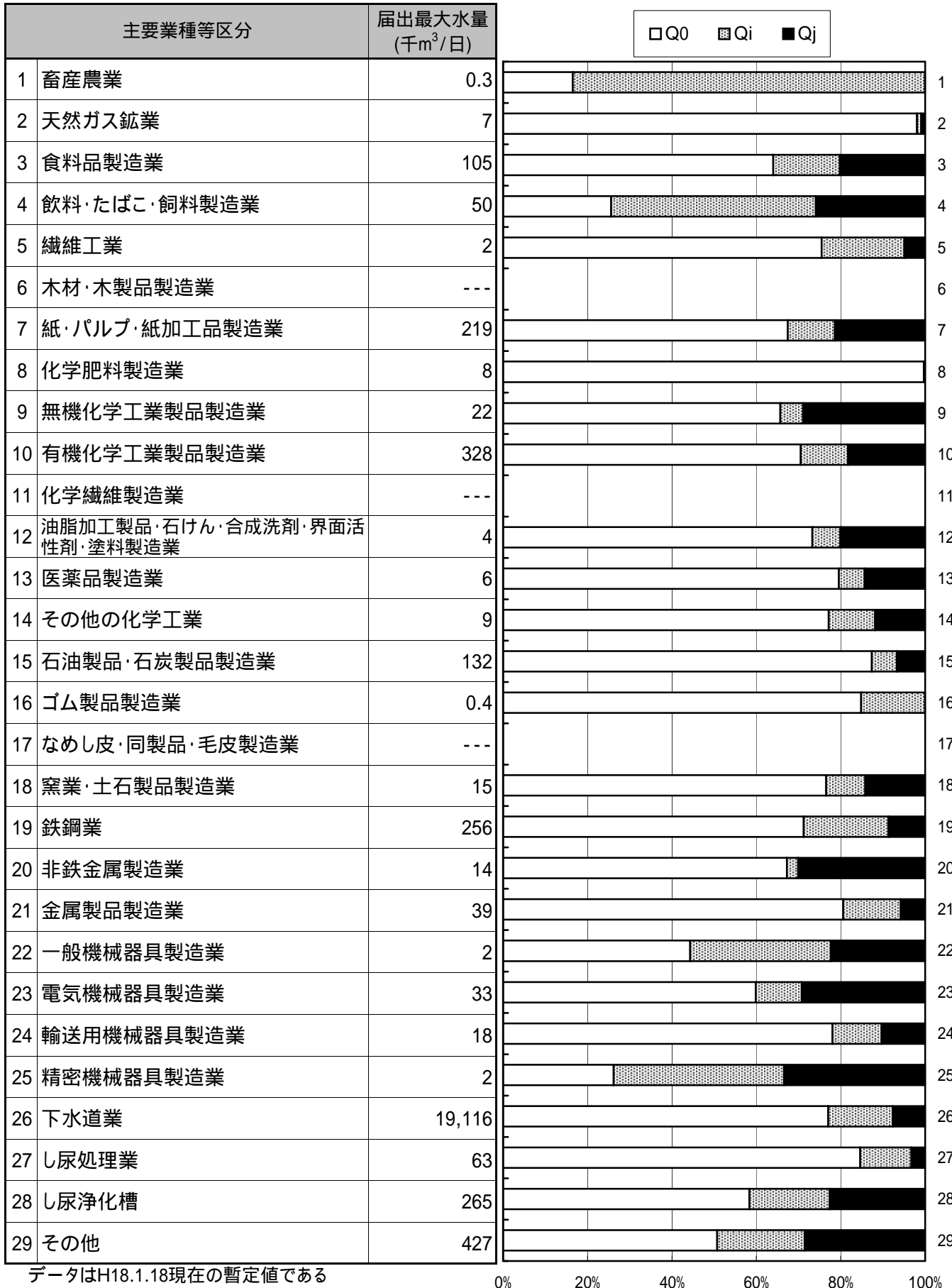
図1-1 東京湾 - COD
