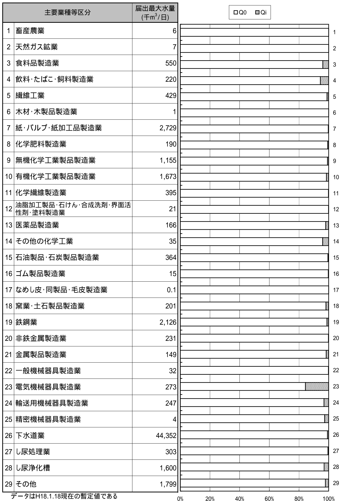
図5 - 2 3海域計 - 窒素・りん
