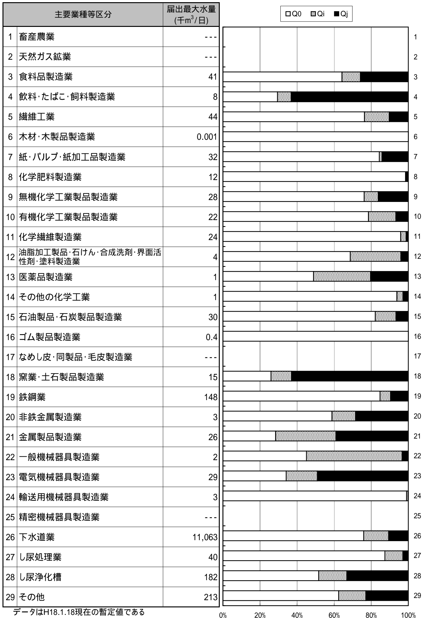
図3 - 1 大阪湾 - COD
