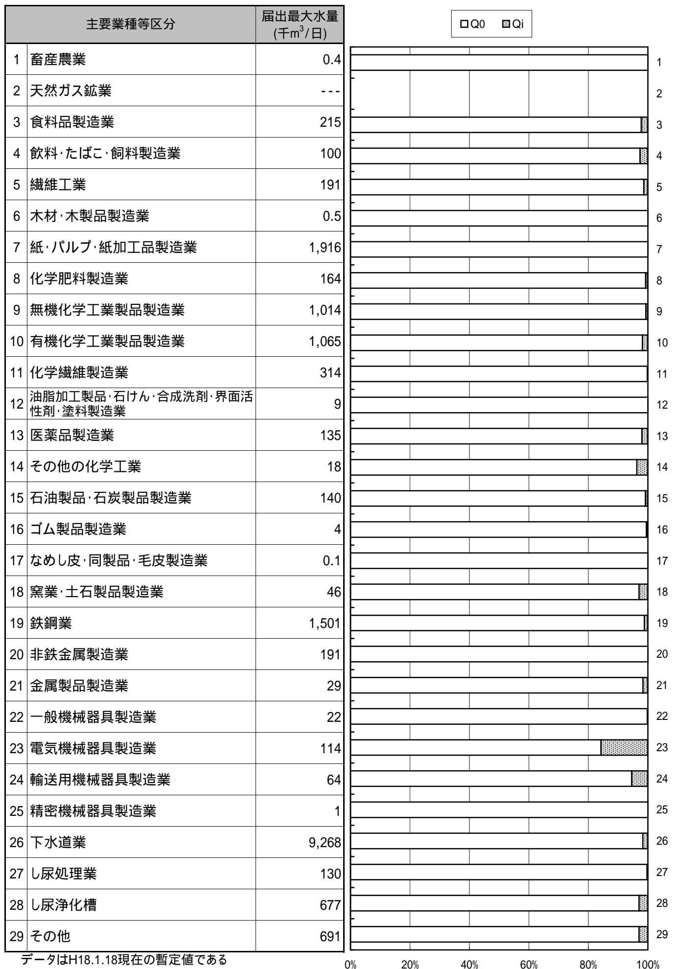
図4 - 2 瀬戸内海（大阪湾除く） - 窒素・りん
