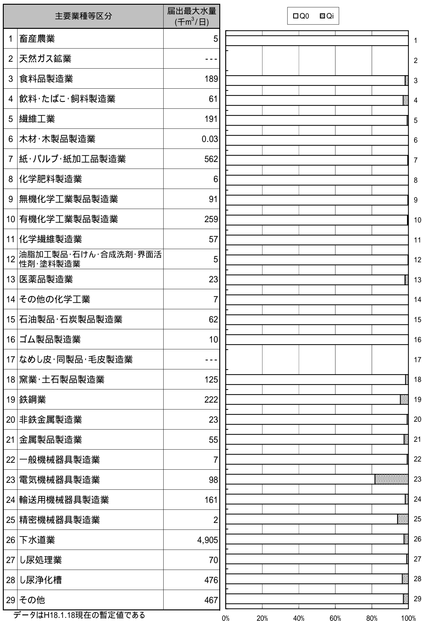
図 2 - 2 伊勢湾 - 窒素・りん
