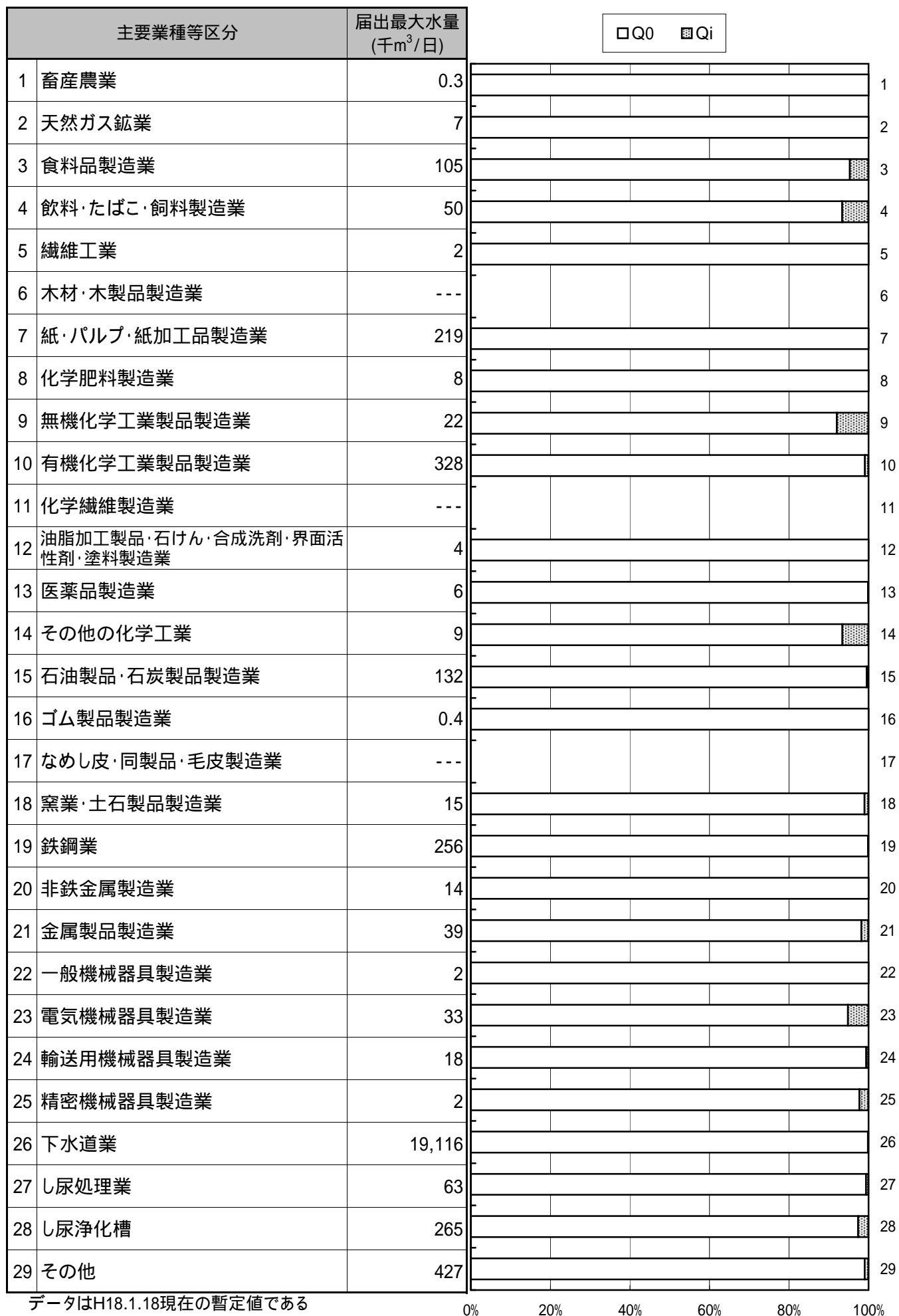
図 1 - 2 東京湾 - 窒素・りん
