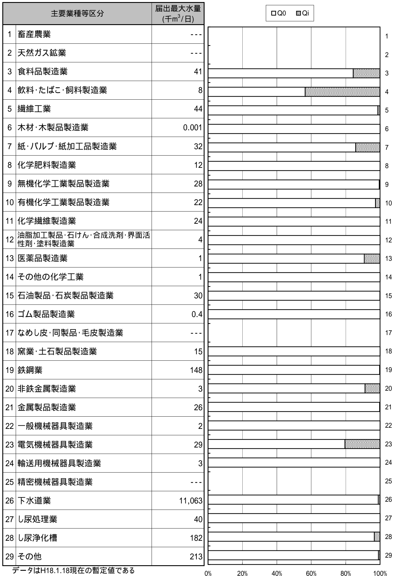
図3 - 2 大阪湾 - 窒素・りん
