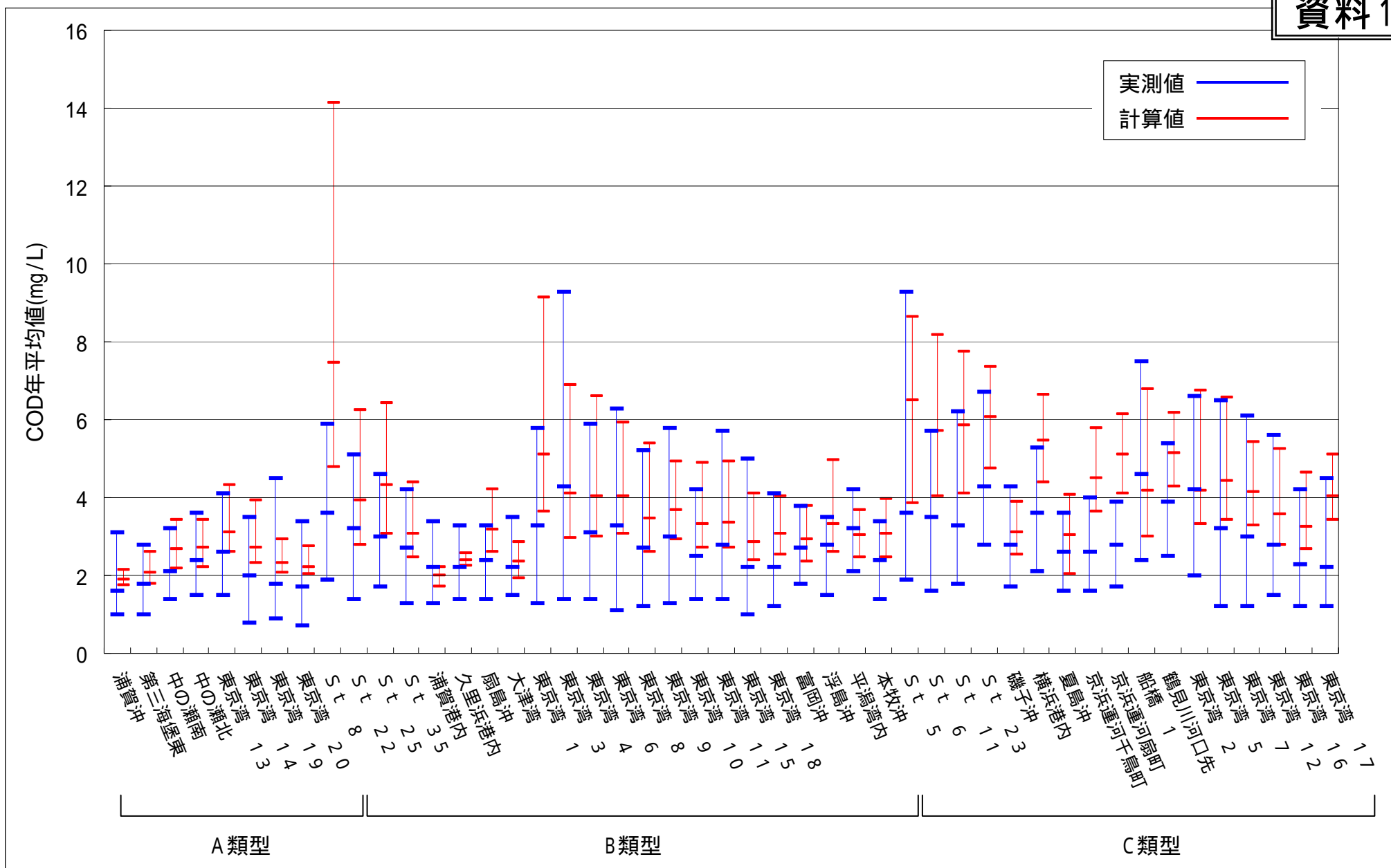
図 - 1 環境基準点における実測値と実測日当日の計算値との比較 (COD)
