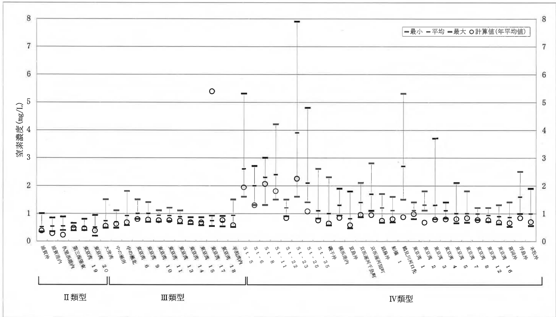
図-4 環境基準点における実測値と計算値の比較(窒素)
