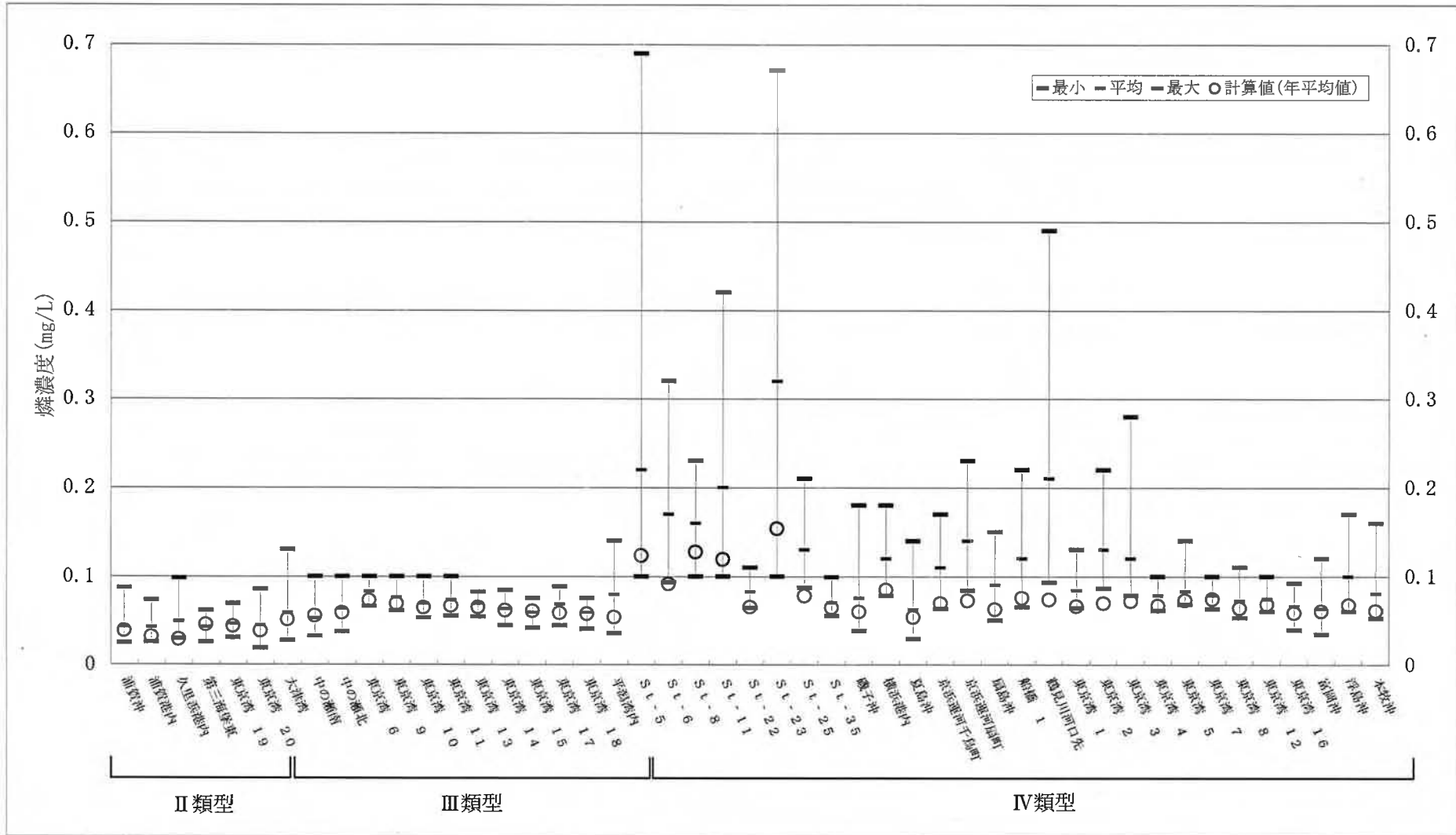
図-5 環境基準点における実測値と計算値の比較(燐)
