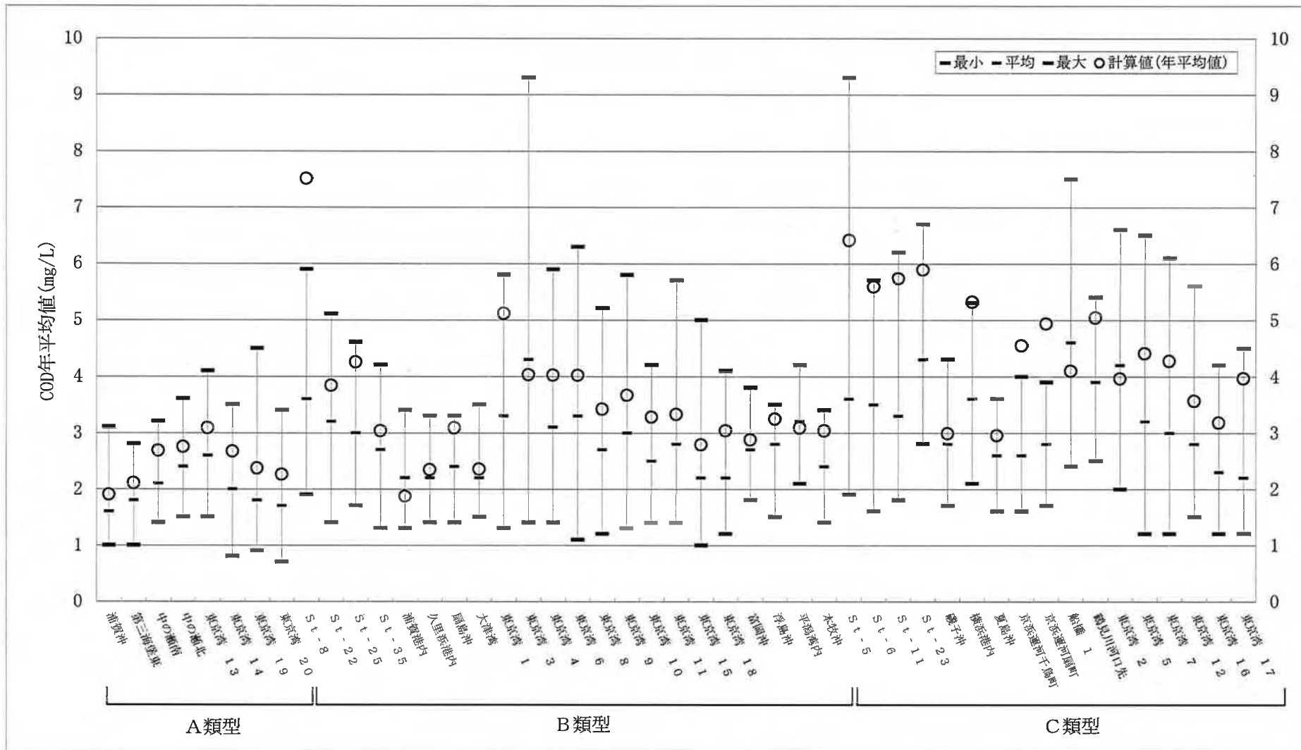
図-3 環境基準点における実測値と計算値の比較(COD)
