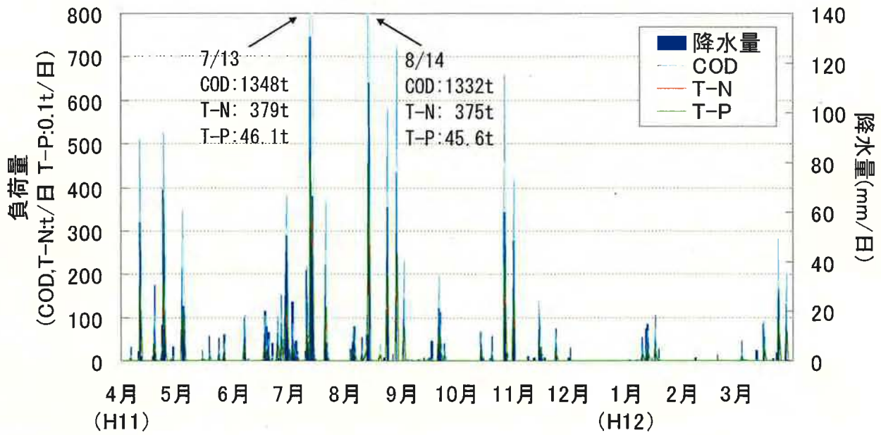
図-5 合流式下水道の雨水吐から越流する負荷量の日変化 D
