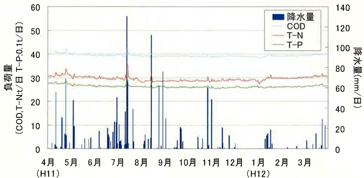
図-4 主要河川以外の河川から海域へ流入する負荷量の日変化 [C]
