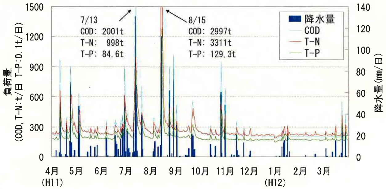
図-7 全負荷量の日変化 (A+B+C+D+E)
