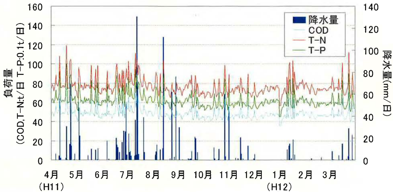
図-3 海域へ直接的に流入する負荷量の日変化 [B]
