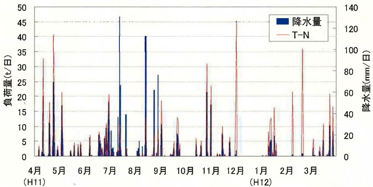
図-6 大気中から直接海域へ流入する負荷量の日変化 E
