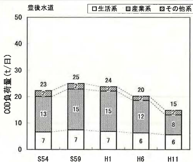
図3. 豊後水道におけるCOD発生負荷量の推移 (出典: 発生負荷量管理等調査)
