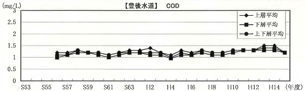
図2. 豊後水道における水質濃度(COD)の推移 (出典: 広域総合水質調査)
