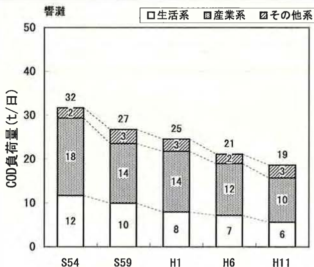
図3. 響灘におけるCOD発生負荷量の推移 (出典:発生負荷量管理等調査)
