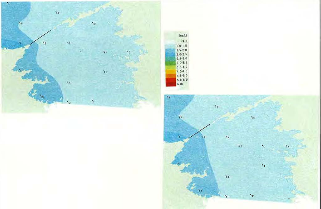
図1. 豊後水道におけるCOD濃度分布(上層3カ年平均 左上: S57~S59年度 右下: H12~H14年度) (出典: 広域総合水質調査)
