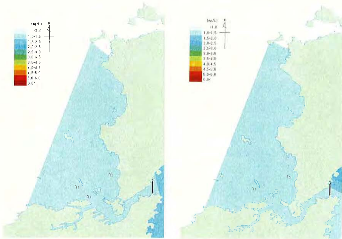
図1. 響灘におけるCOD濃度分布(上層3年平均 左:S57~S59年度 右:H12~H14年度) (出典:広域総合水質調査)
