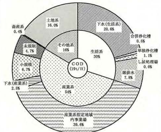
図4. 響灘のCOD発生源別発生負荷量 (平成11年度) (出典:発生負荷量管理等調査)
