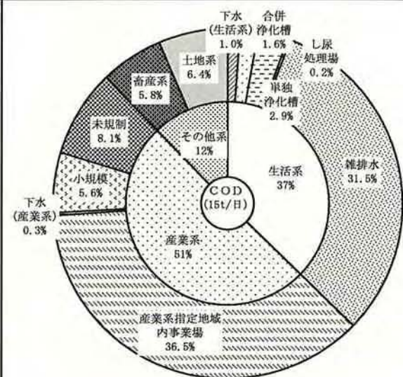
図4. 豊後水道のCOD発生源別発生負荷量 (平成11年度) (出典: 発生負荷量管理等調査)
