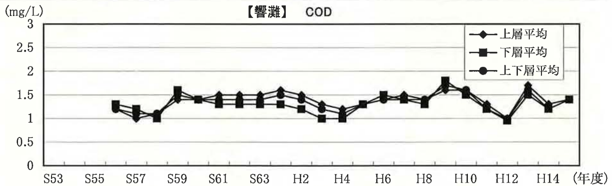
図2. 響灘における水質濃度(COD)の推移 (出典:広域総合水質調査)
