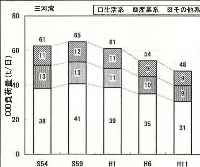
図3. 三河湾におけるCOD発生負荷量の推移 (出典: 発生負荷量管理等調査)
