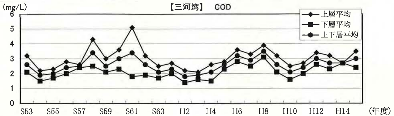
図2. 三河湾における水質濃度(COD)の推移 (出典: 広域総合水質調査)
