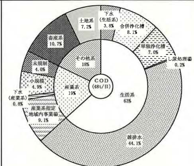
図4. 三河湾のCOD発生源別発生負荷量 (平成11年度) (出典: 発生負荷量管理等調査)
