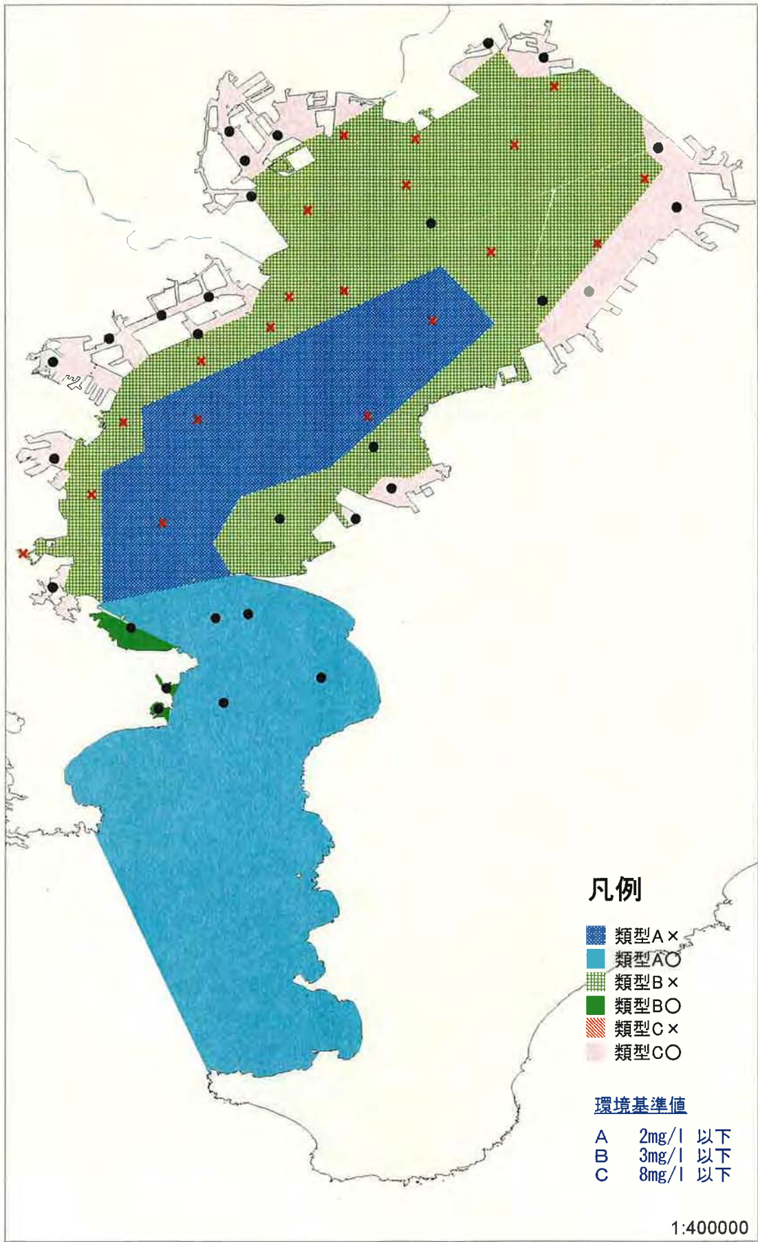
COD環境基準値の適合状況 東京湾 (平成14年度)
