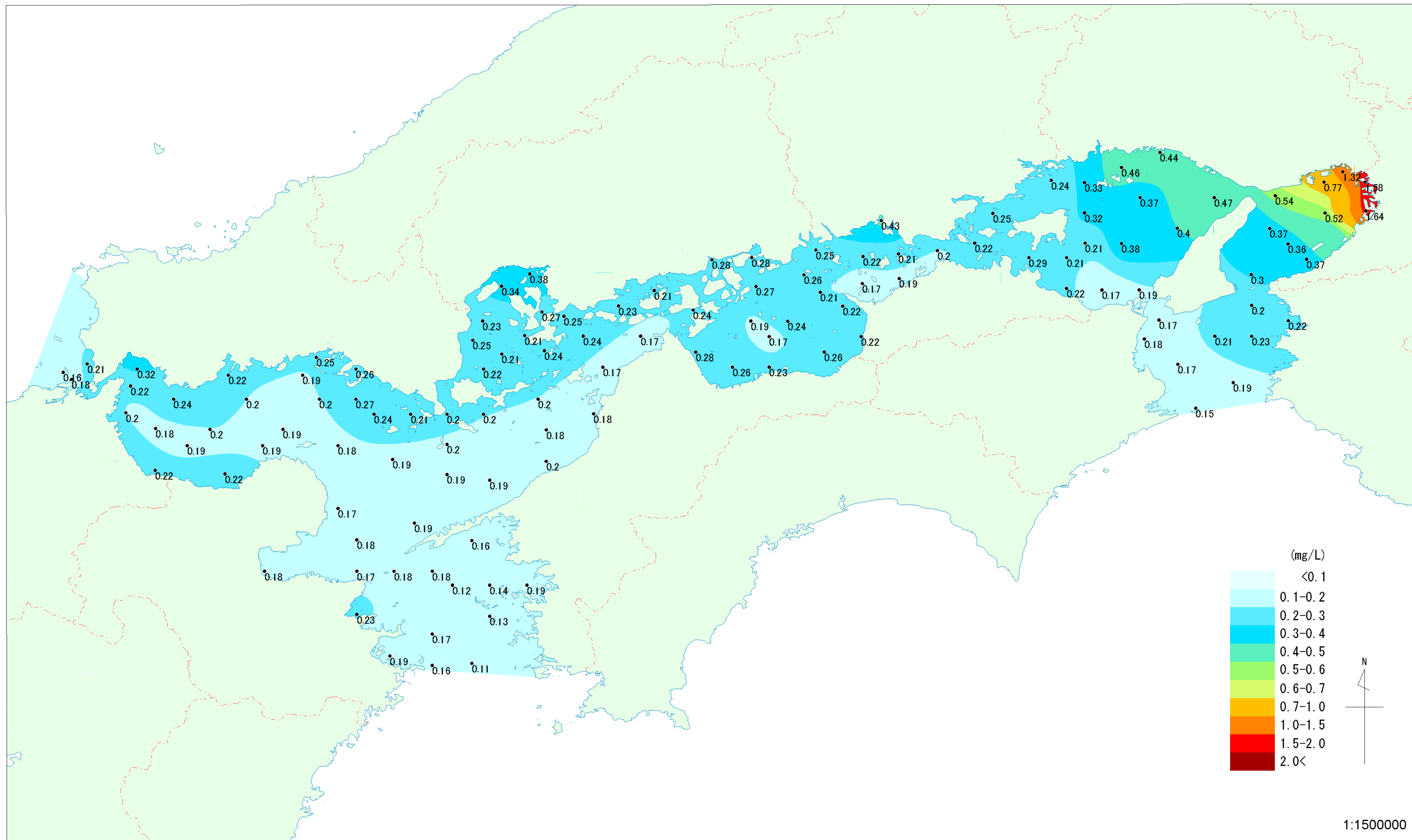
瀬戸内海におけるT-Nの分布 (2000~2002年度 上層・3ヵ年平均)
