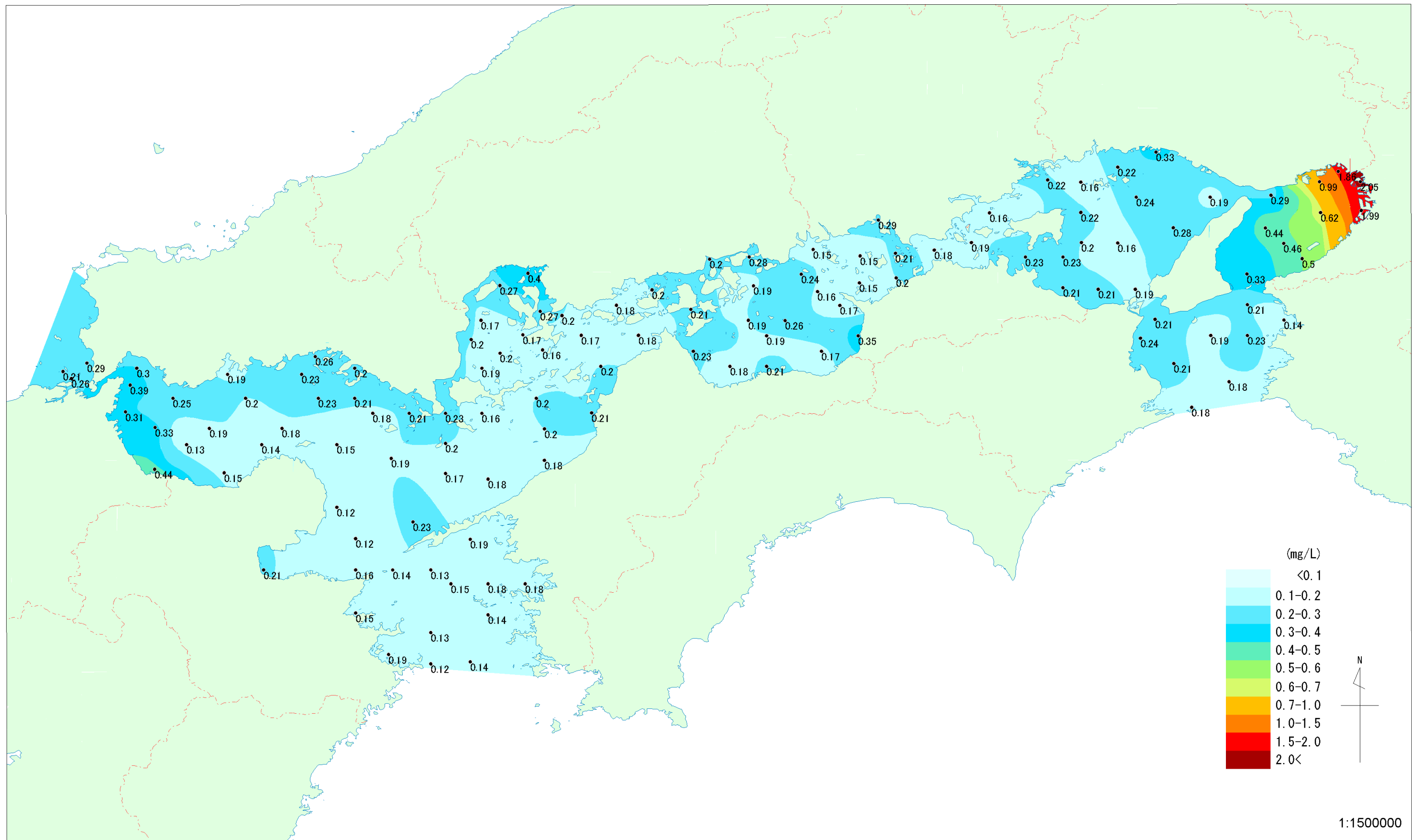
瀬戸内海におけるT-Nの分布 (1982~1984年度 上層・3ヵ年平均)
