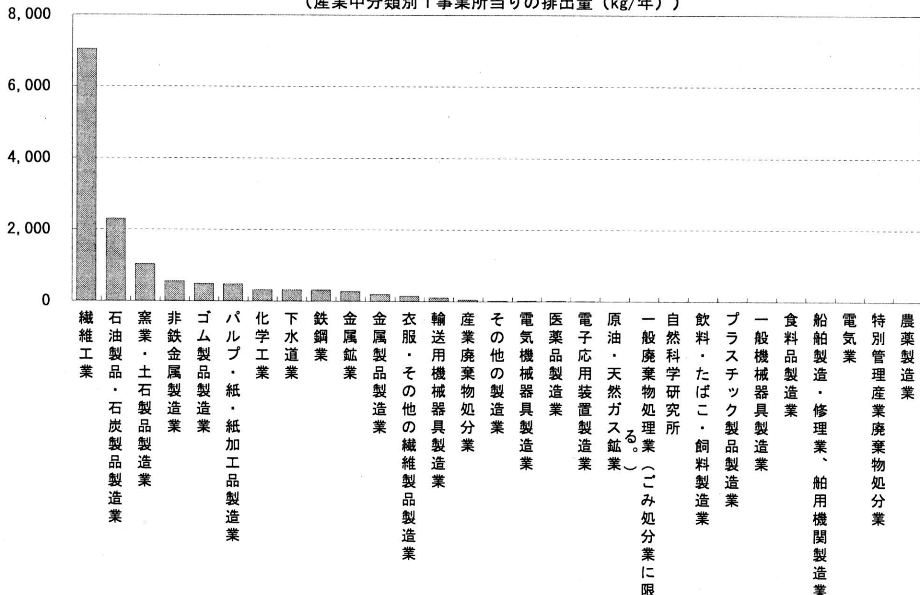
PRTRデータに基づく水溶性亜鉛の公共用水域排出状況 (産業中分類別1事業所当りの排出量 (kg/年))
