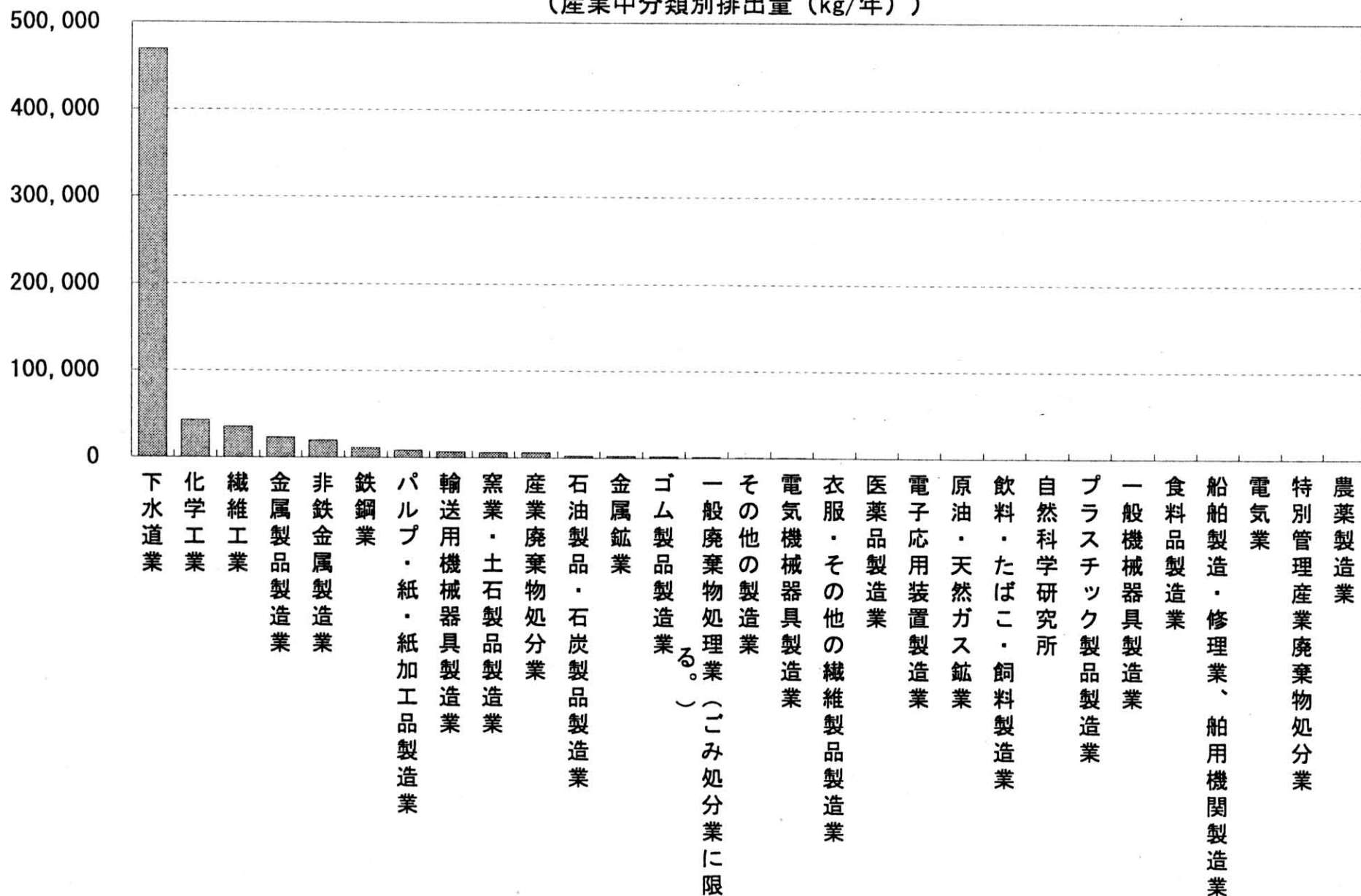
PRTRデータに基づく水溶性亜鉛の公共用水域排出状況 (産業中分類別排出量 (kg/年))
