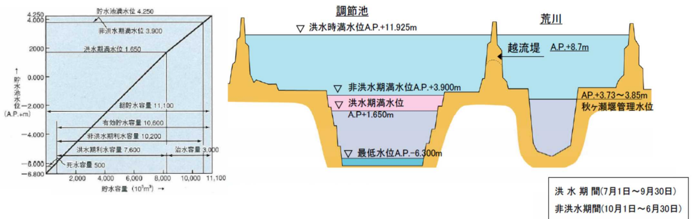
図 2-1 荒川貯水池（彩湖）貯水容量配分図
