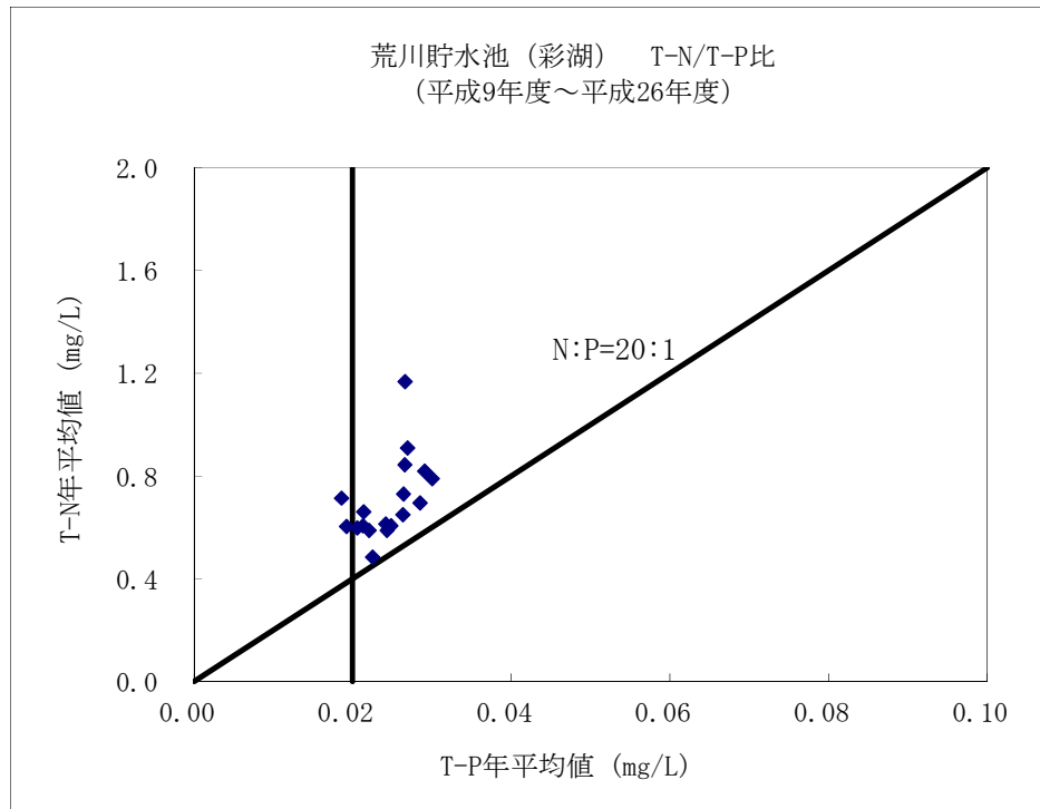
図 2-7 荒川貯水池（彩湖）N/P比の状況
