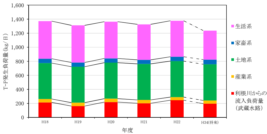
図 2-20 荒川貯水池（彩湖）流域の T-P 汚濁負荷量経年変化
