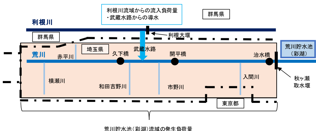
図 2-16 荒川貯水池（彩湖）への水質汚濁負荷量の流入概念図
