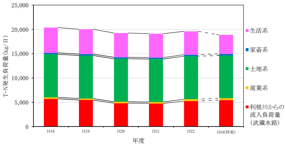
図 2-19 荒川貯水池（彩湖）流域の T-N 汚濁負荷量経年変化
