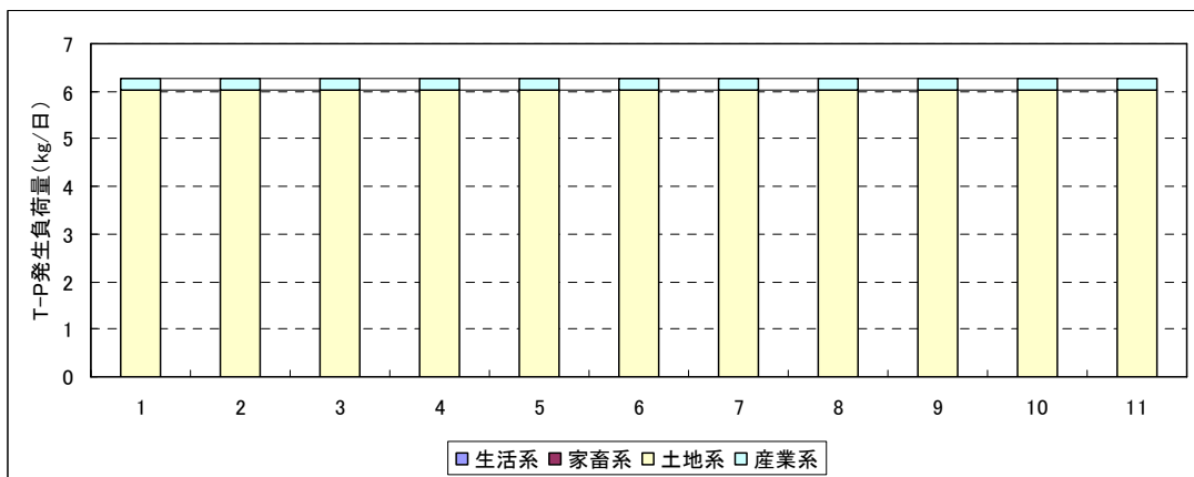
图 3.14 T-P 発生負荷量経年変化
