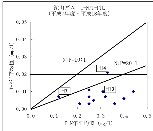
図 3.6 深山ダム N/P 比の状況
