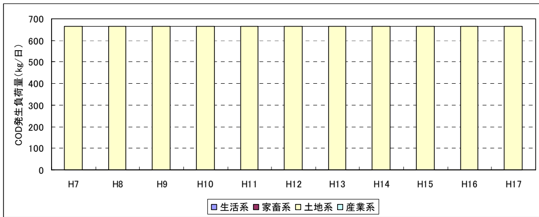
图 3.12 COD 発生負荷量経年変化
