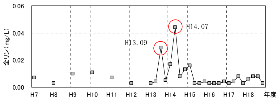
図 3.7 深山ダム全リン経月変化
