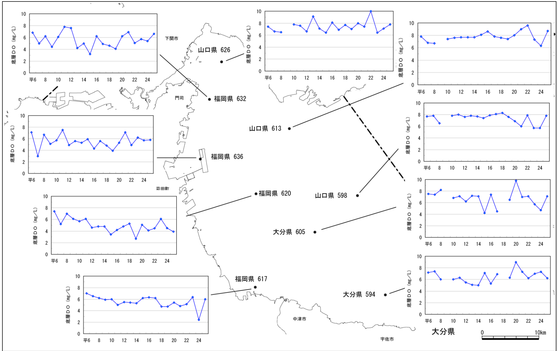
図 3.13 周防灘南西岸における夏季の底層DO濃度の推移
