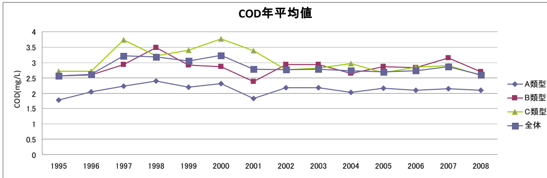
図6.3 CODの推移
