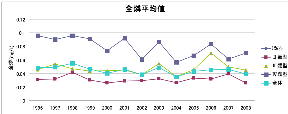
図6.5 全燐の推移
