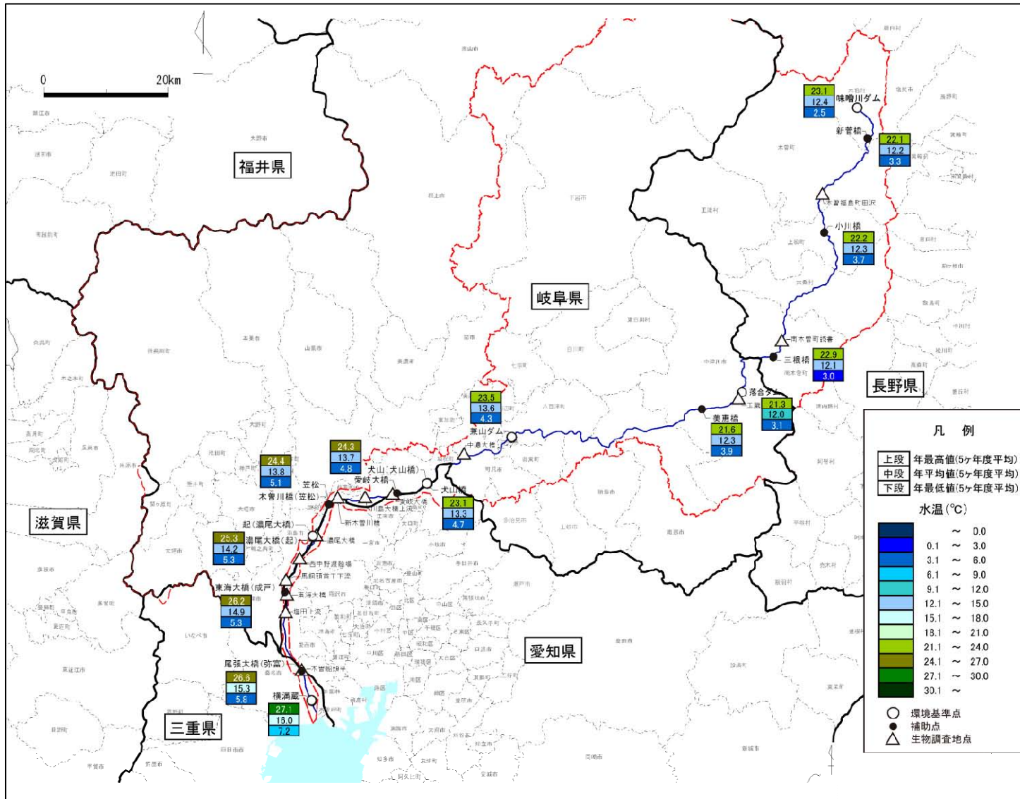
図 4.8 水温(木曾川)
