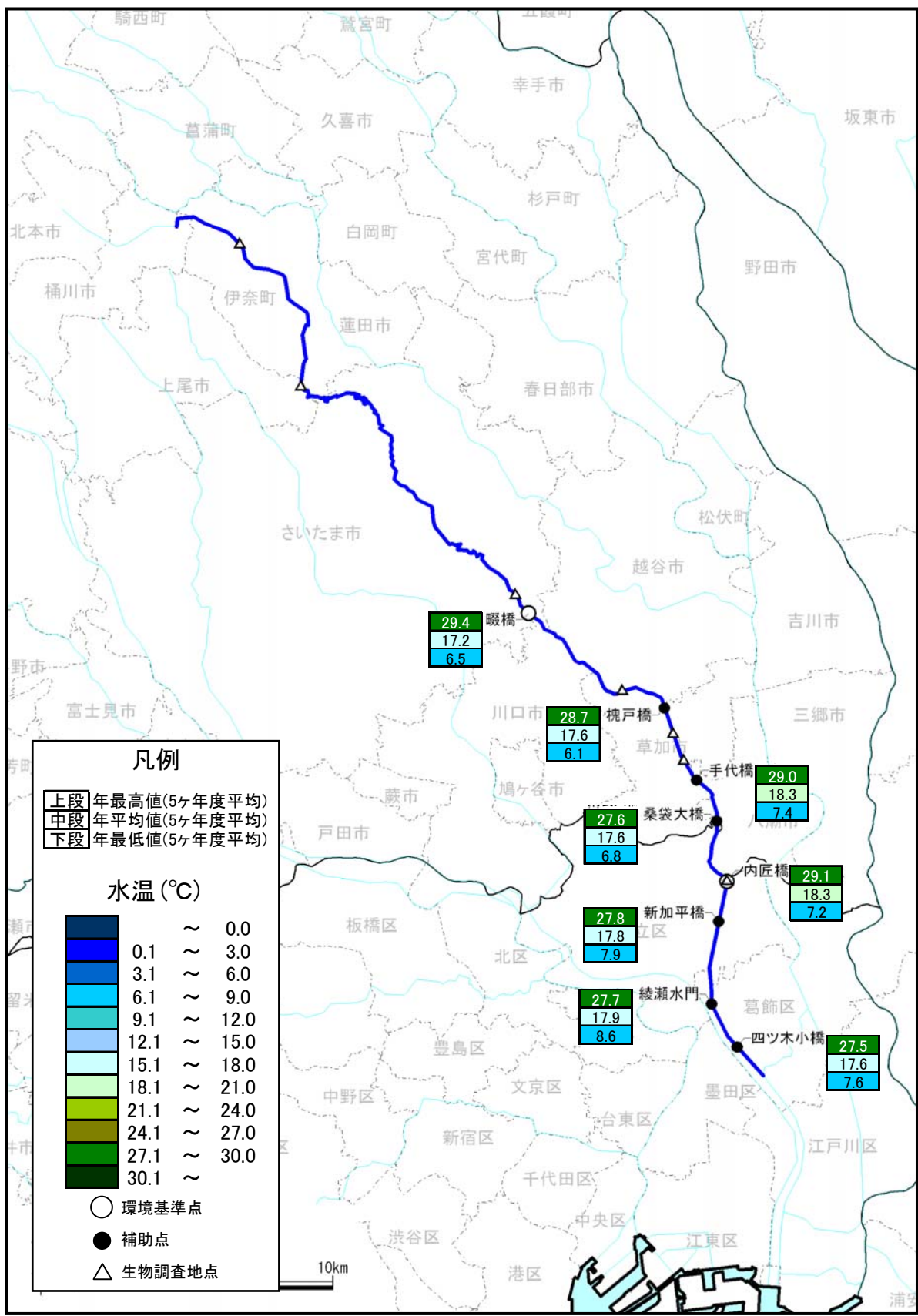
図5.6 綾瀬川【水温】
