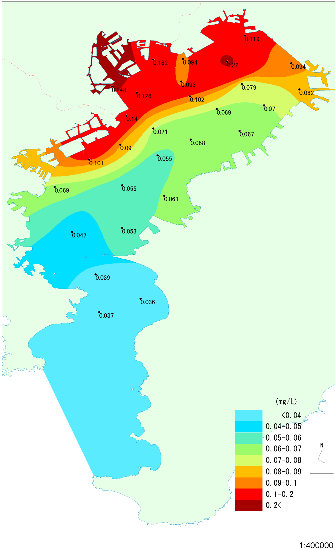
東京湾におけるT-Pの分布 (2000~2002年度 上層・3カ年平均)
