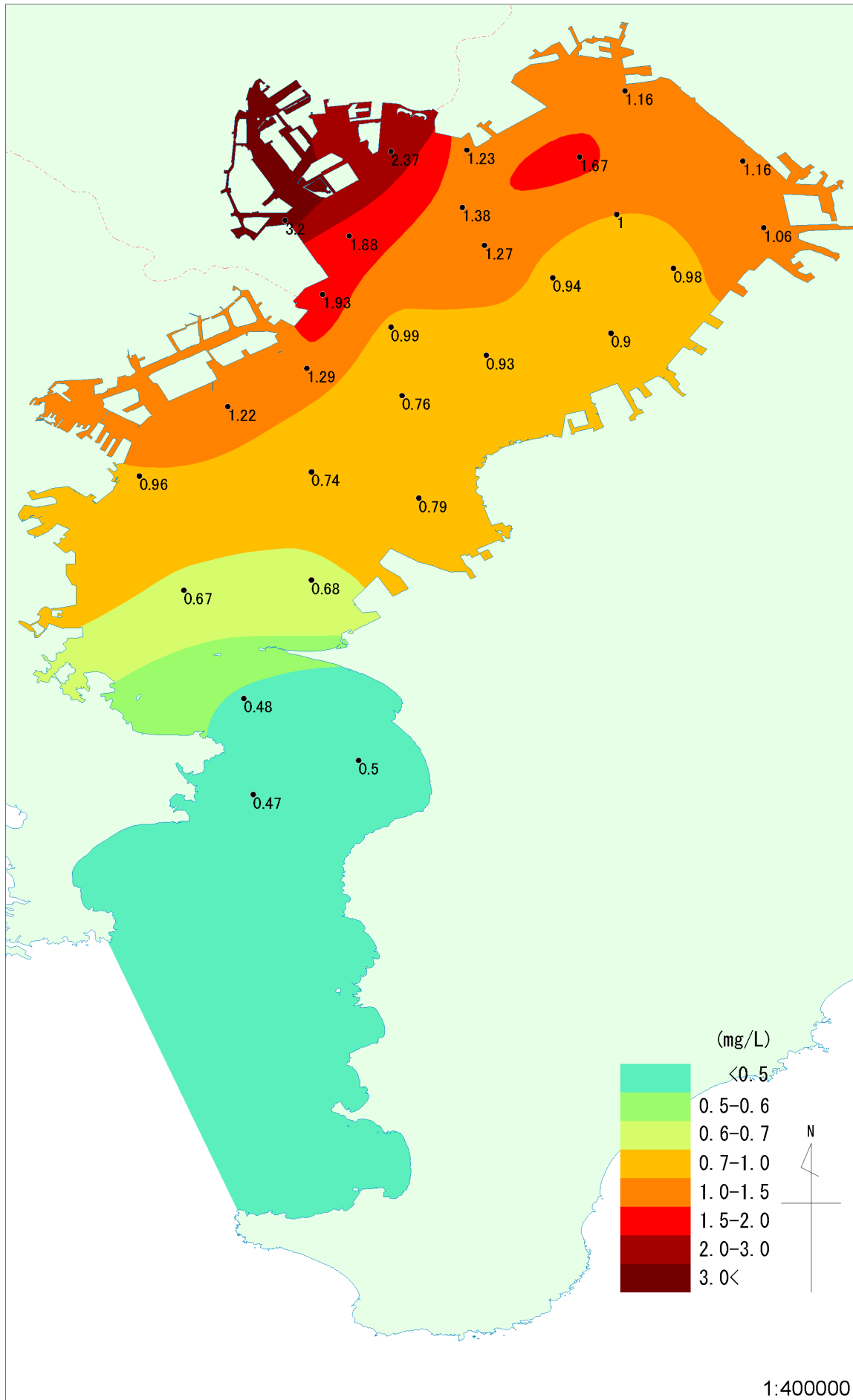
東京湾におけるT-Nの分布 (2000~2002年度 上層・3カ年平均)
