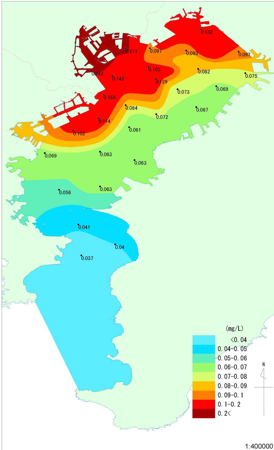
東京湾におけるT-Pの分布 (1982~1984年度 上層・3カ年平均)
