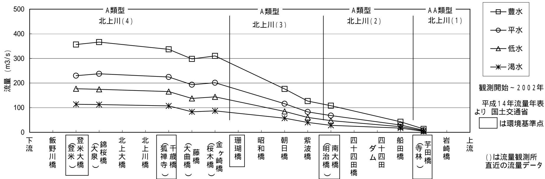
図3.1.10 流量の縦断分布
