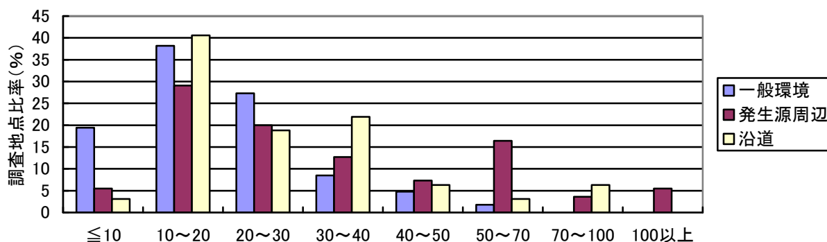
図3 20112010年度のマンガンに係る有害大気汚染物質モニタリング調査結果の濃度分布
