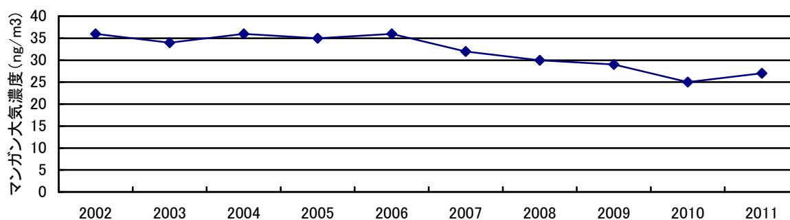
図2 有害大気汚染物質モニタリング調査の継続調査地点 (142 地点) のマンガン及びその化合物の年平均濃度の推移
