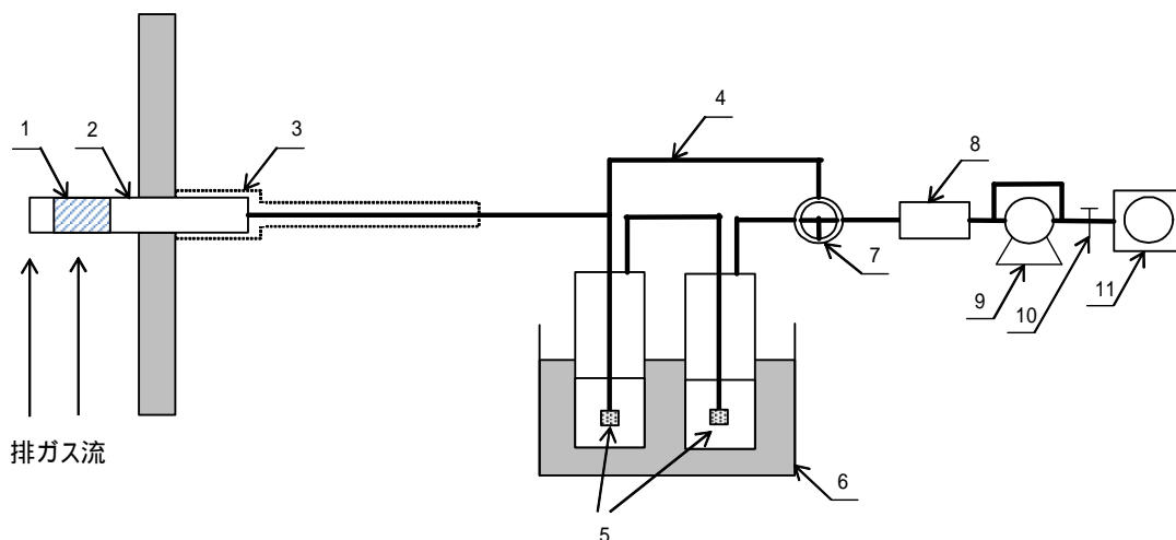
図 試料採取装置の構成（一例）
