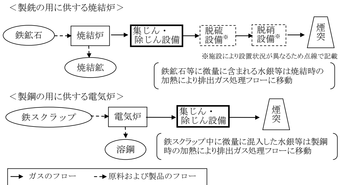
図4 要排出抑制施設におけるフローの一例
