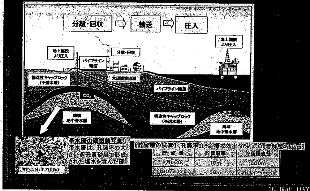
図2-2 地中貯留の概念図
