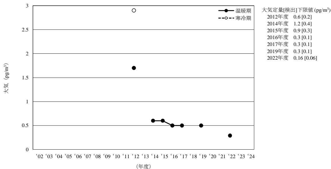
[19-1] \alpha -1,2,5,6,9,10-ヘキサブロモシクロデカン
