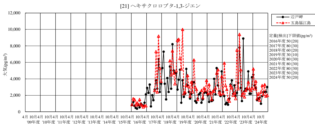
図 18 ヘキサクロブタ-1,3-ジエンの経月変化
