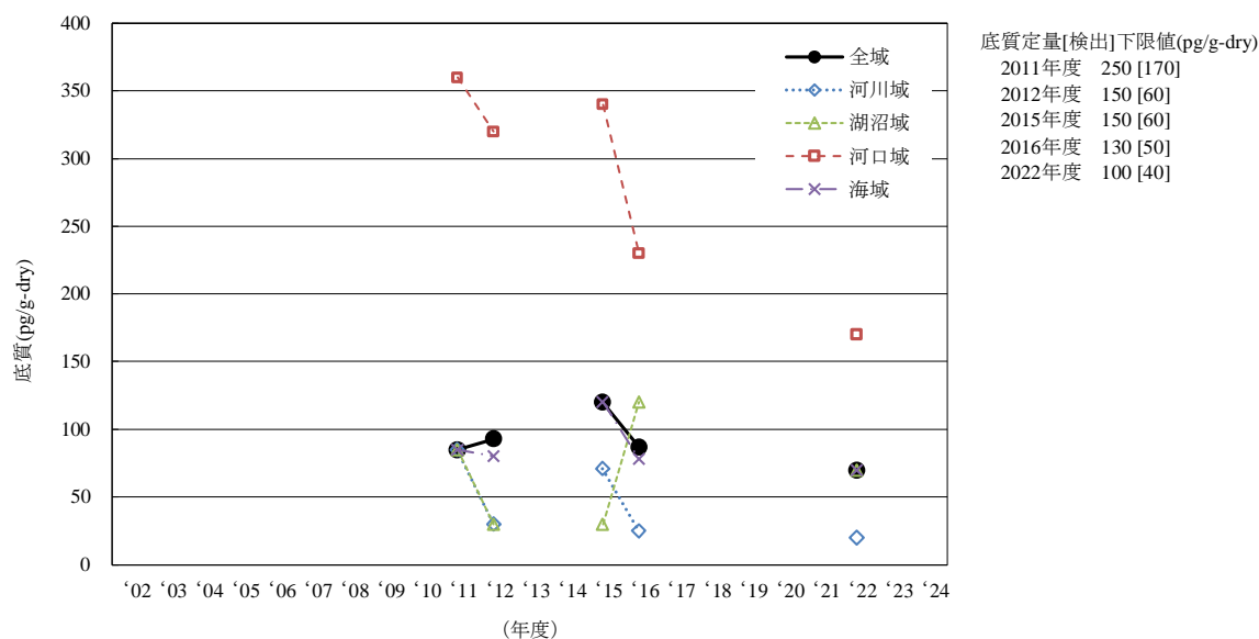
[19-2] \beta -1,2,5,6,9,10-ヘキサブロモシクロデカン
