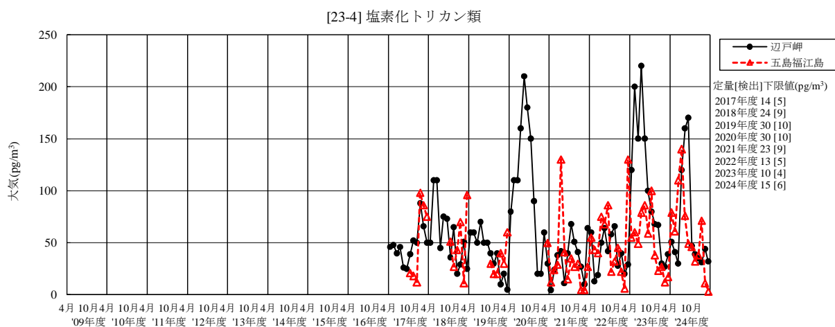
図 20-4 塩素化トリデカン類の経月変化
