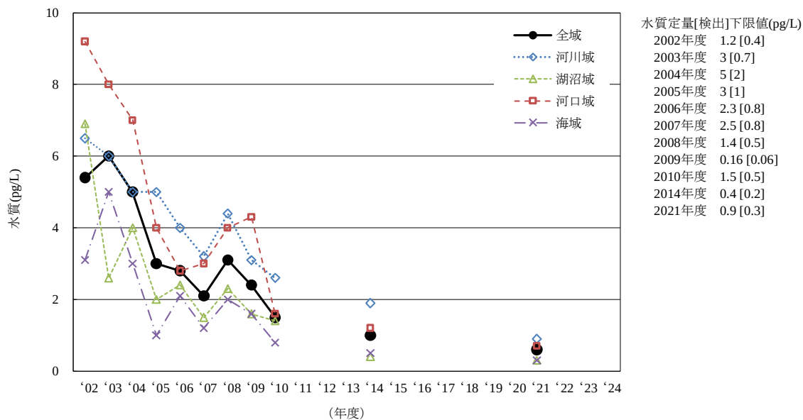
[6-4] o,p' -DDT
