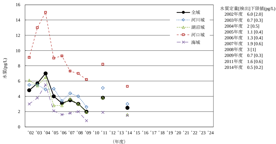
[5] エンドリン
