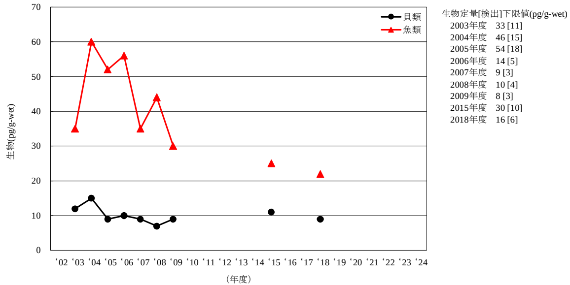
[9-2] Parlar-50
