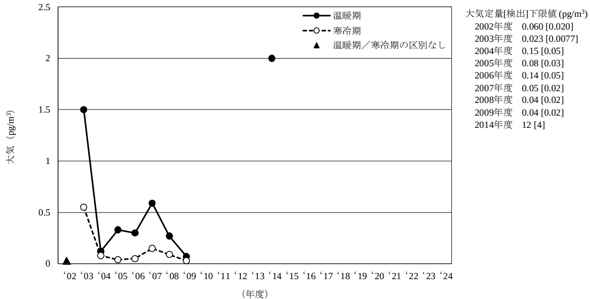
[3] アルドリン
