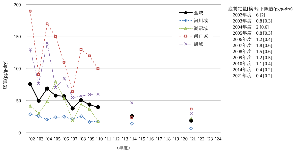
[6-4] o,p' -DDT
