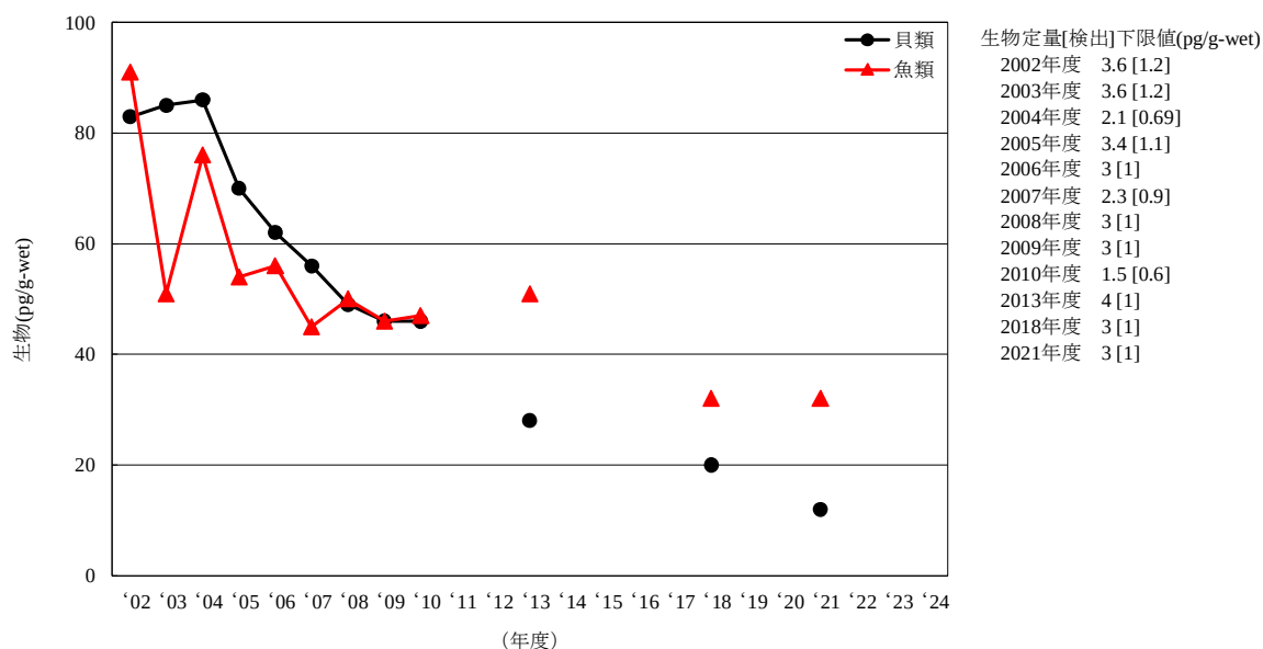
[6-5] o,p' -DDE
