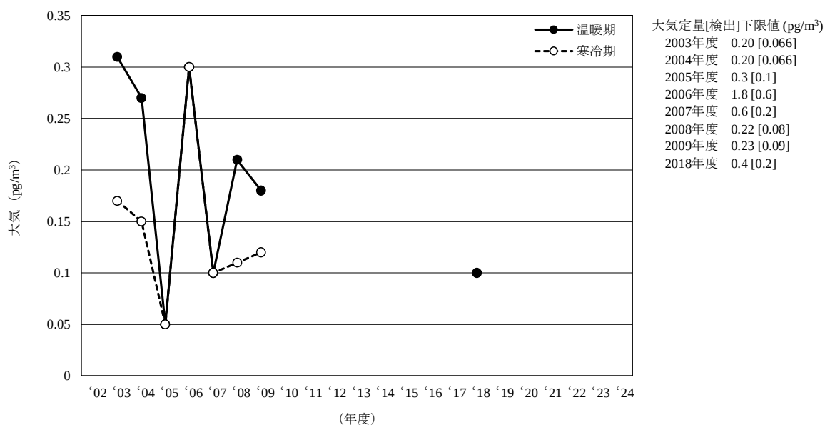
[9-1] Parlar-26
