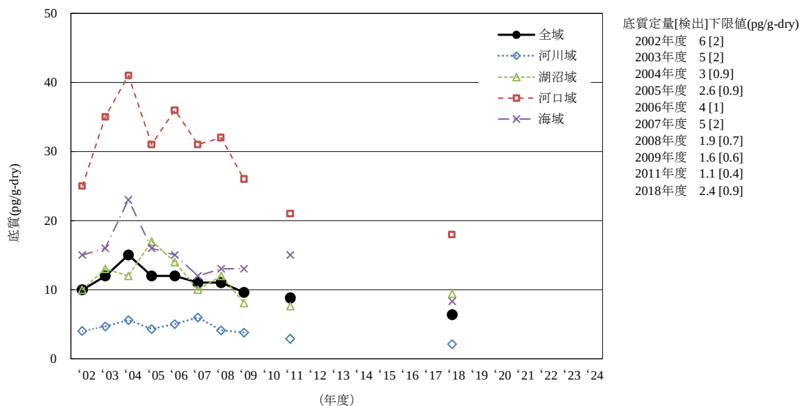
[5] エンドリン
