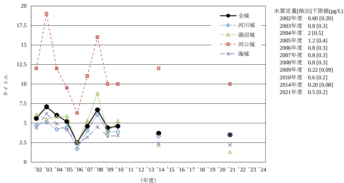
[6-6] o,p' -DDD
