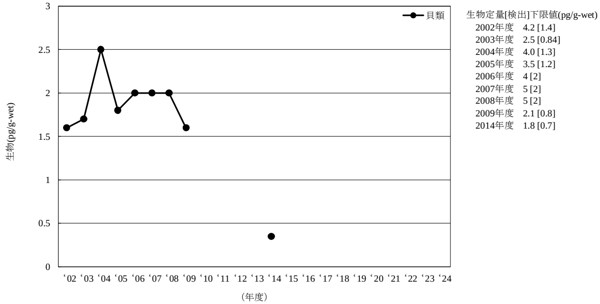
[3] アルドリン
