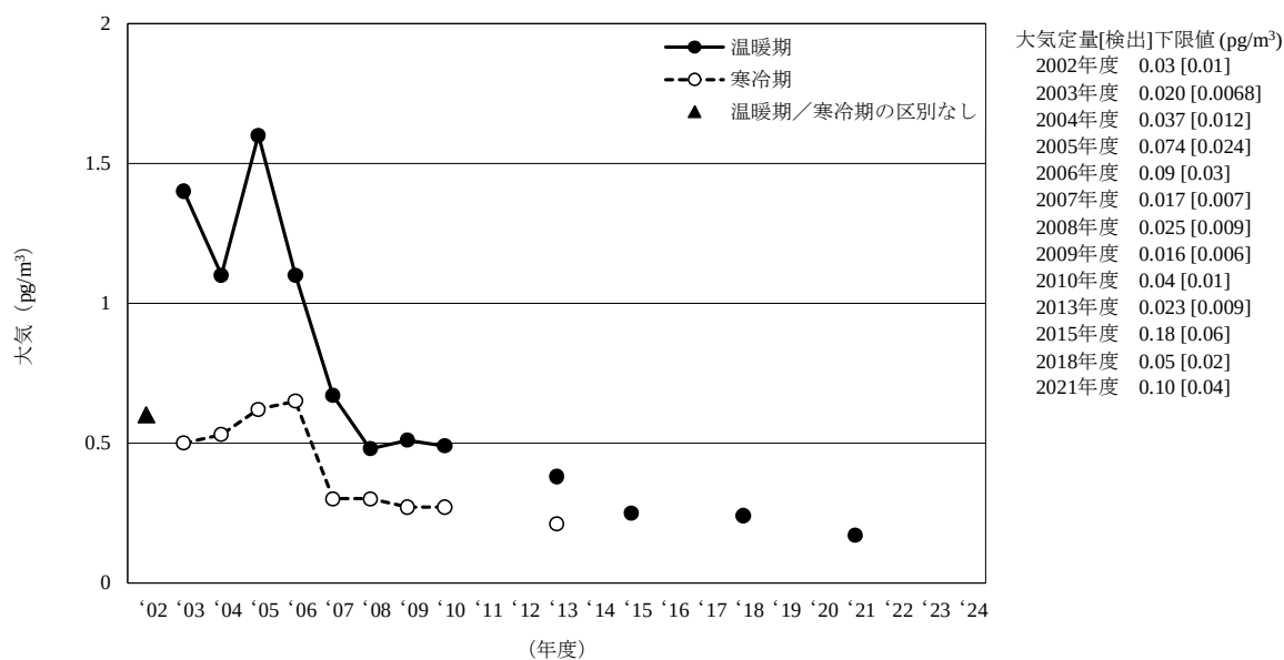
[6-5] o,p' -DDE
