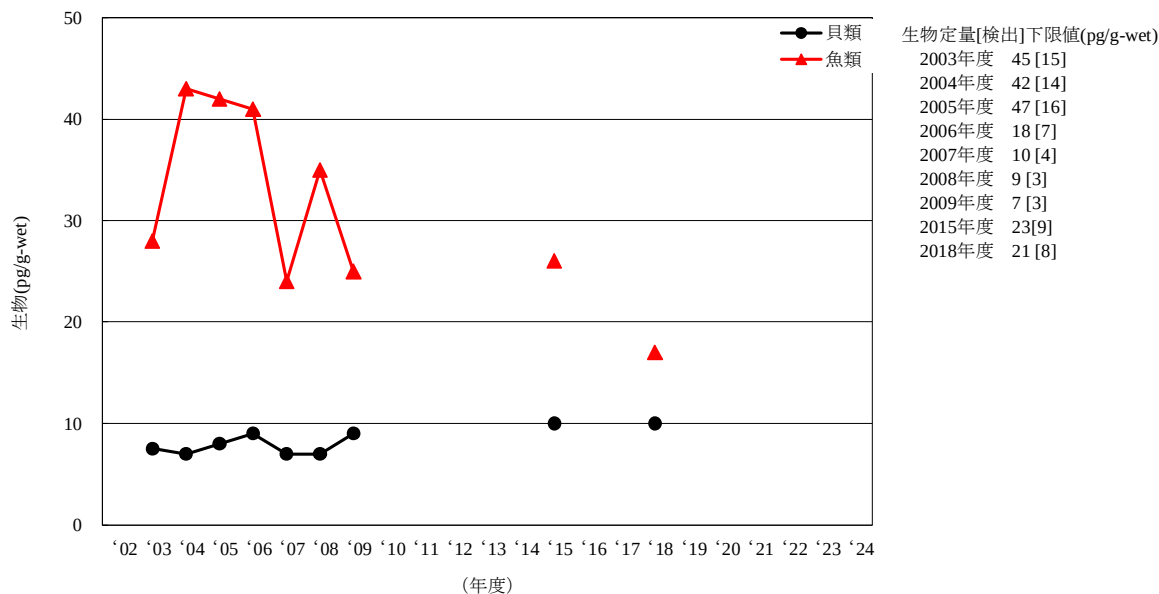
[9-1] Parlar-26
