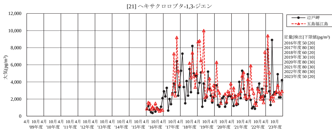
図 18 ヘキサクロブタ-1,3-ジエンの経月変化
