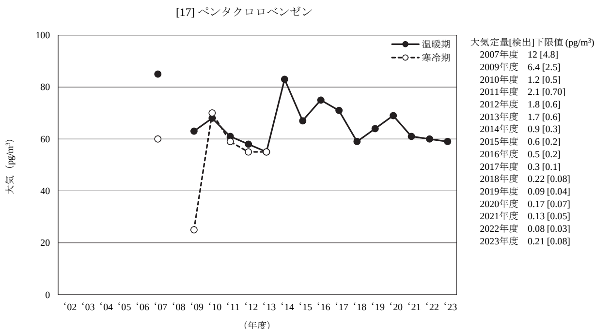
図 3-17-2 ペンタクロロベンゼンの大気の経年変化（幾何平均値）
