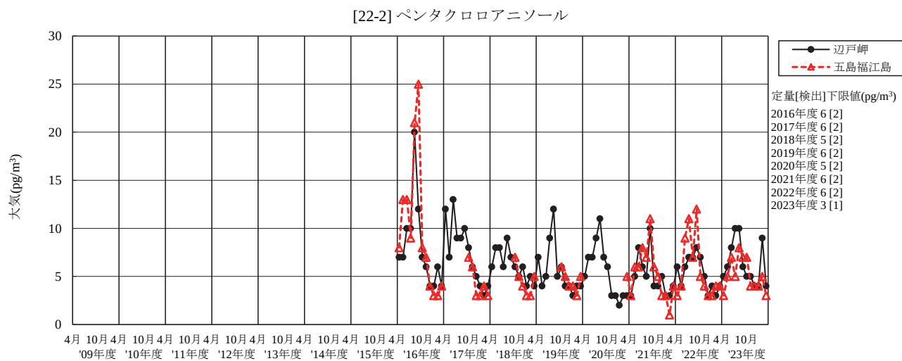
図 19-2 ペンタクロロアニソールの経月変化
