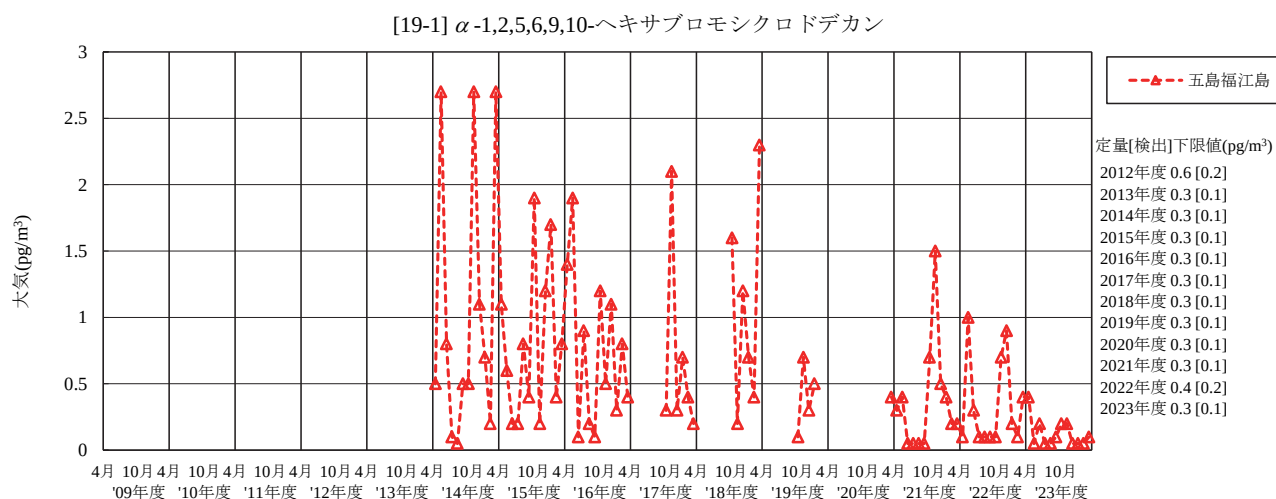
図 16-1 \alpha -1,2,5,6,9,10-ヘキサブロモシクロデカンの経月変化
