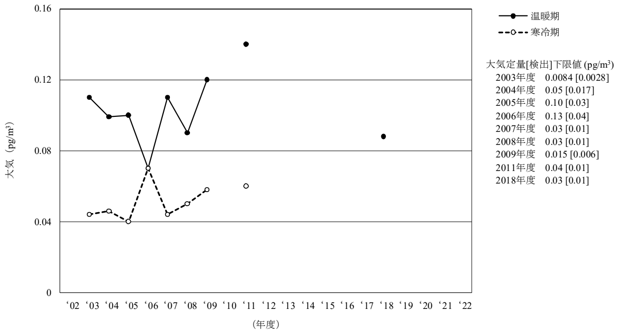
図 3-10-4 マイレックスの大気の時年変化 (幾何平均値)
