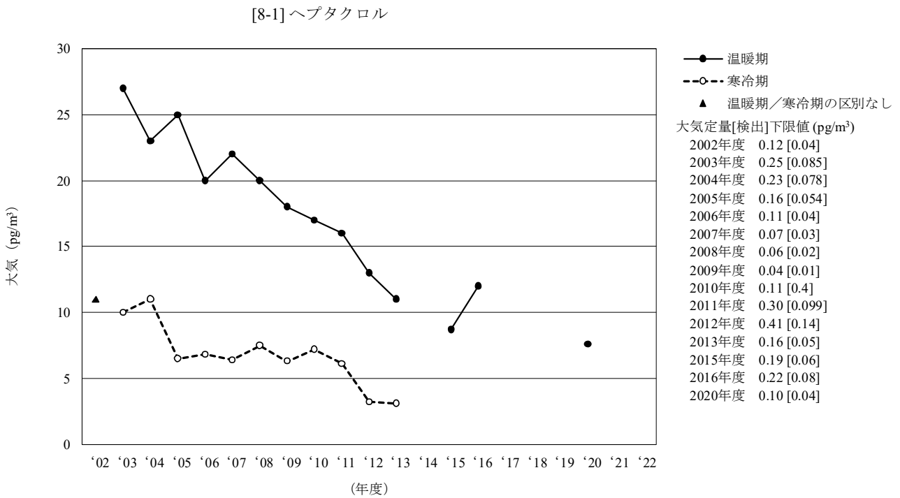
図3-8-1-2 ヘプタクロルの大気の大気経年変化（幾何平均値）
