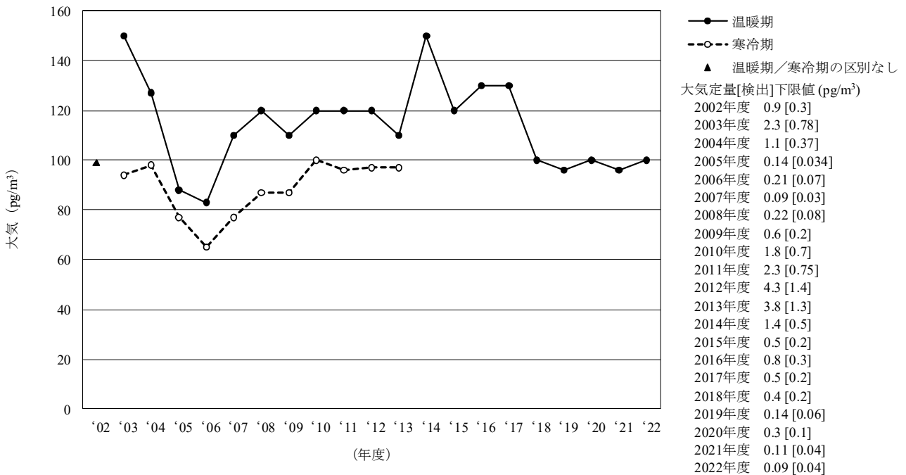
図 3-2-4 HCB の大気の大気経年変化 (幾何平均値)
