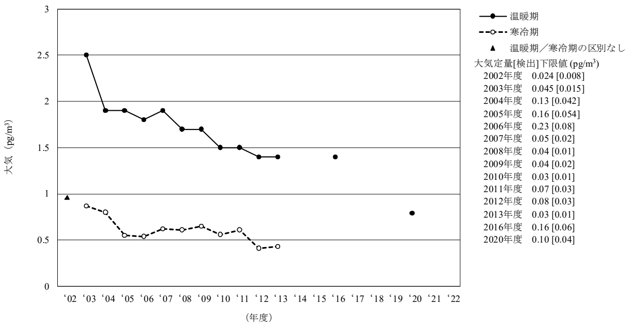
図 3-7-3-4 オキシクロルデンの大気の大気経年変化（幾何平均値）
