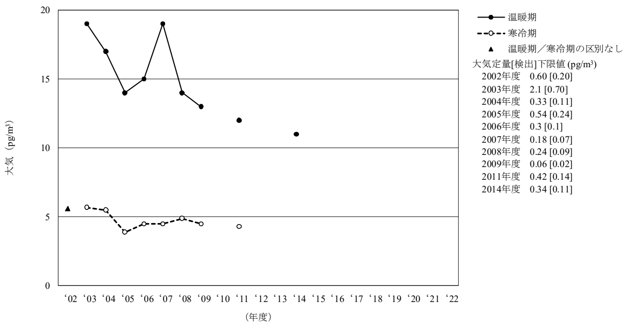
図 3-4-4 ディルドリンの大気の大気の経年変化 (幾何平均値)
