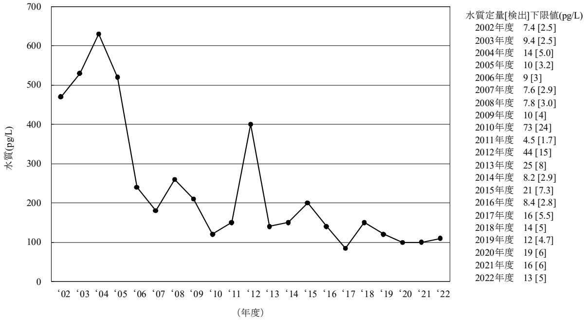
[1] 総PCB
