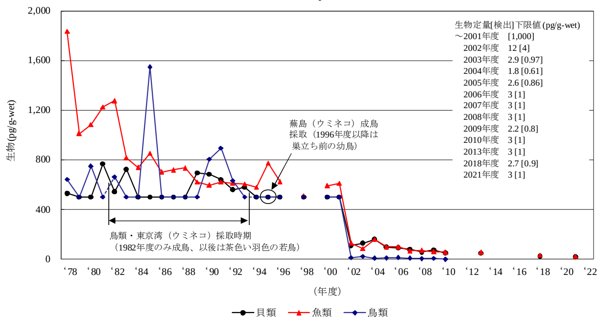
[6-4] o,p' -DDT
