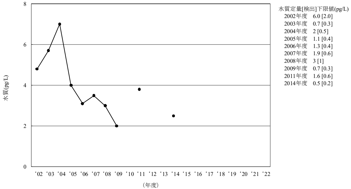
[5] エンドリン
