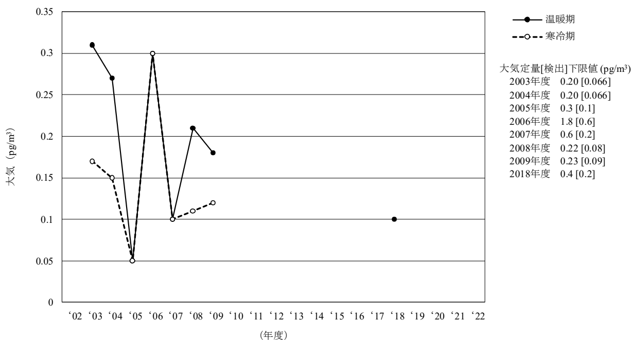
[9-1] Parlar-26
