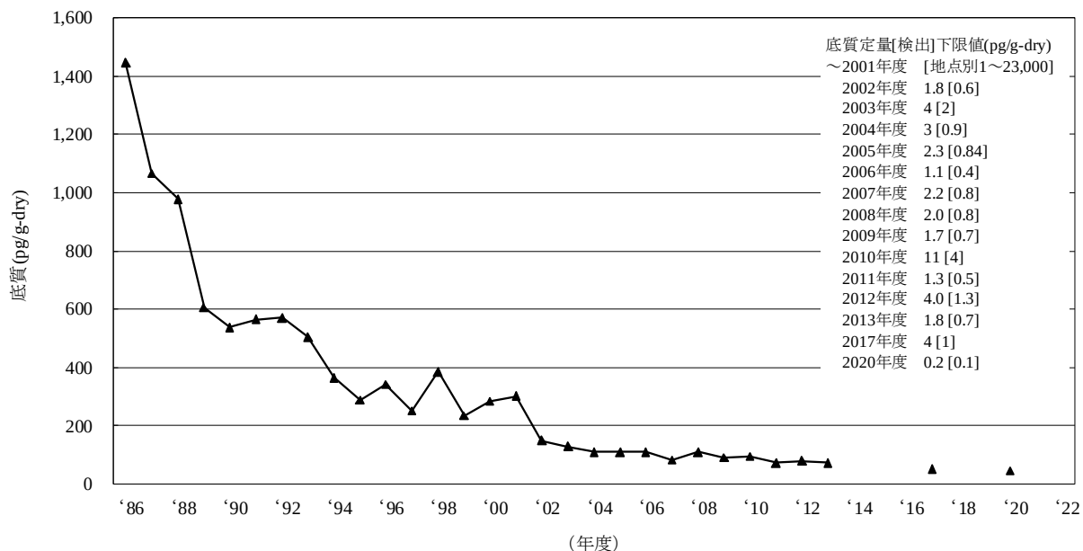
図 6-2-1 trans -クロルデンの底質の経年変化 (幾何平均値)
