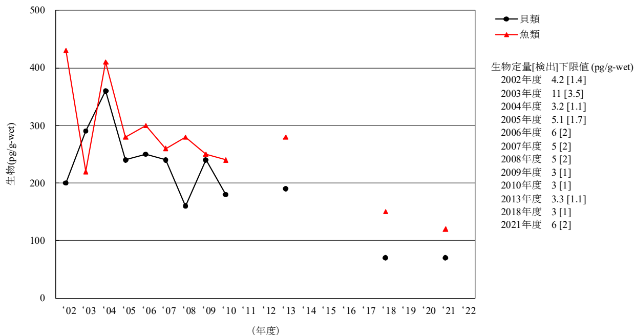
[6-1] p,p' -DDT
