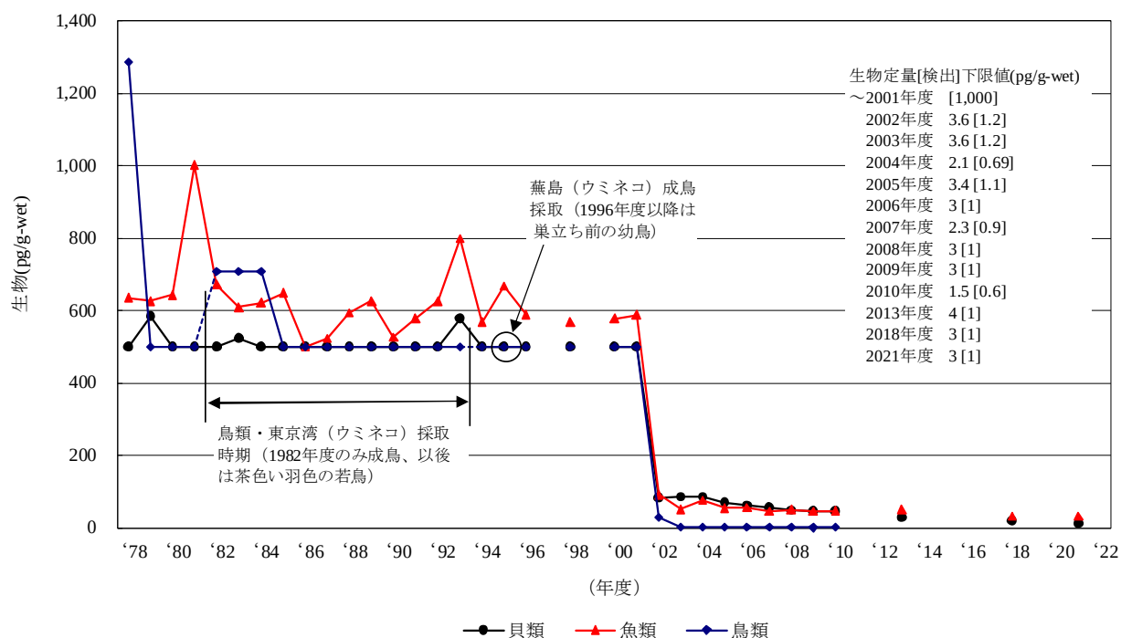
[6-5] o,p' -DDE
